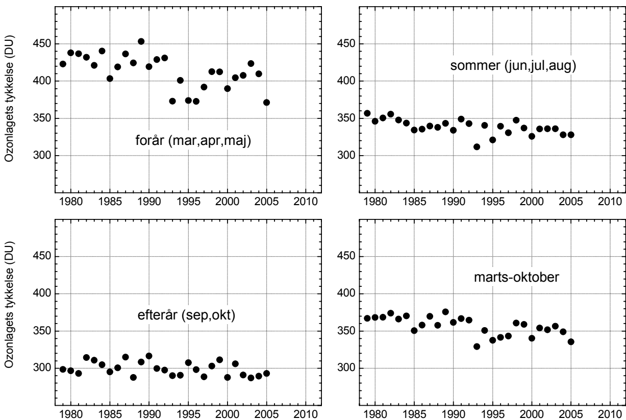
Figur 9. Ozonlagets sæsonmæssige middeldykkelse for Kangerlussuaq for perioden 1979-2005. Der kan kun måles i perioden fra midt i februar til slutningen af oktober. Efterår er derfor begrænset til to måneder, og den årlige middeldykkelse kan ikke bestemmes. En simpel lineær tilpasning af data for perioden 1979-2005 viser en signifikant nedadgående tendens for forår, sommer og hele måleperioden, men ikke for efteråret. Data fra før 1991 er data fra NASA's TOM-instrument på Nimbus-7-satellitten, mens data fra og med 1991 er DMI's målinger med et Brewer-instrument.
