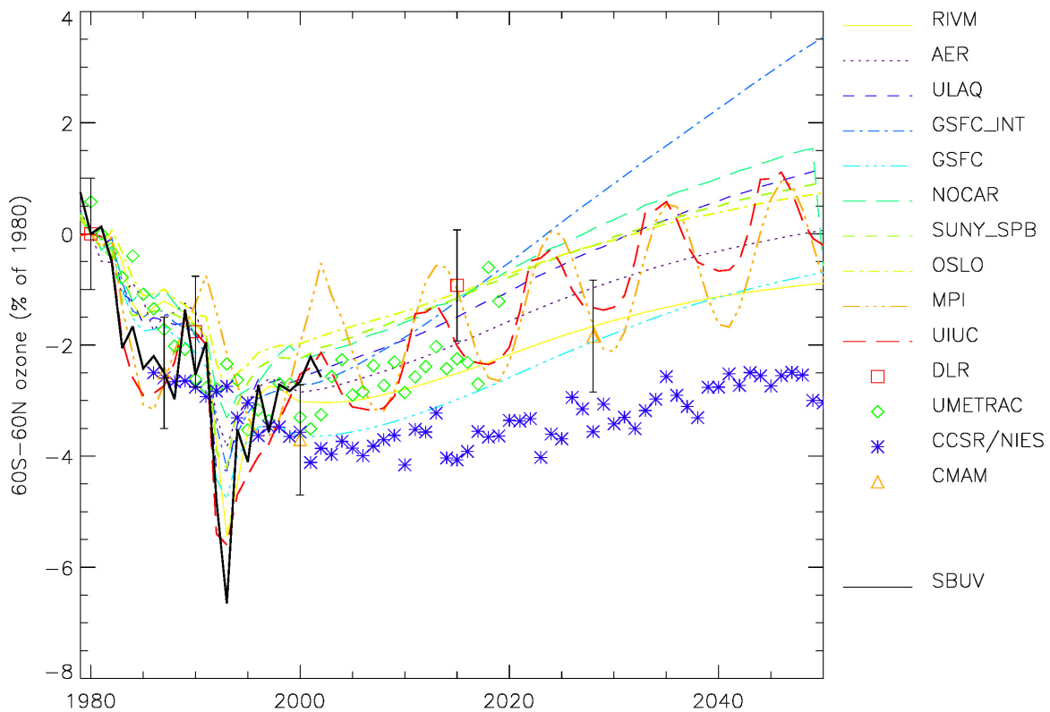
Figur 31. Modelforudsigelser af fremtidens ozonlag midlet fra 60°S til 60°N. De stiplede linier viser resultaterne fra to-dimensionelle modeller, symbolerne fra tre-dimensionelle modeller, og den fuldt optrukne sorte linie er satellitobservationer. De meget lave værdier omkring 1993 skyldes udbruddet af vulkanen Mount Pinatubo på Filippinerne.
