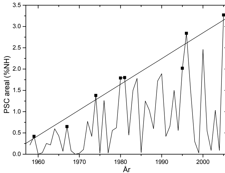
Figur 22. Det gennemsnitlige areal af polar-stratosfæriske skyer i procent af den nordlige halvkugles areal siden 1958. Vintrene med de største PSC-arealer er markeret med kvadrater og danner grundlaget for regressionslinien.
