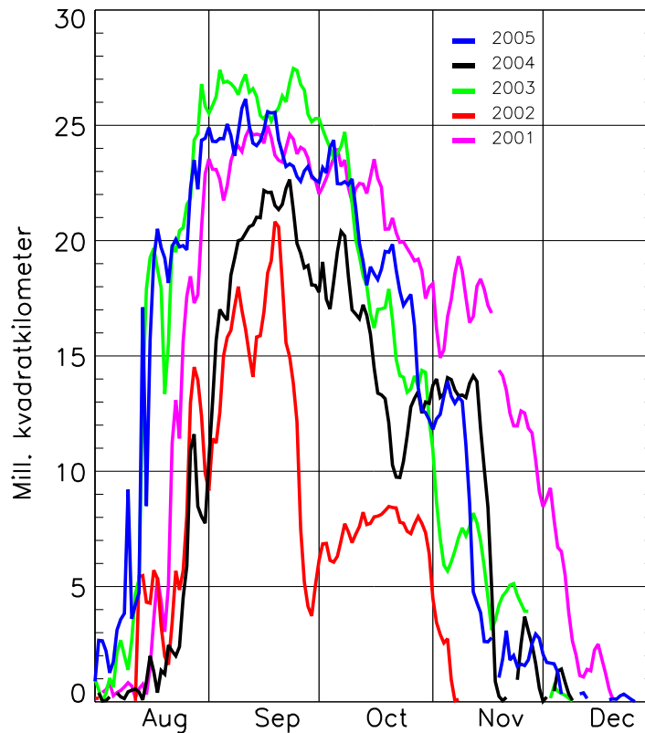
Figur 29. Udviklingen i det antarktiske ozonhuls areal de seneste 5 år.
