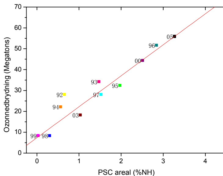
Figur 23. Den maksimale ozonnedbrydning fra januar til marts i den arktiske hvirvel fra 1992-2000 samt 2003 og 2005 som funktion af vinterens gennemsnitlige PSC-areal. Punktet for 1992 er influeret af store mængder af aerosoller fra Pinatubo vulkanens udbrud i juni 1991.
