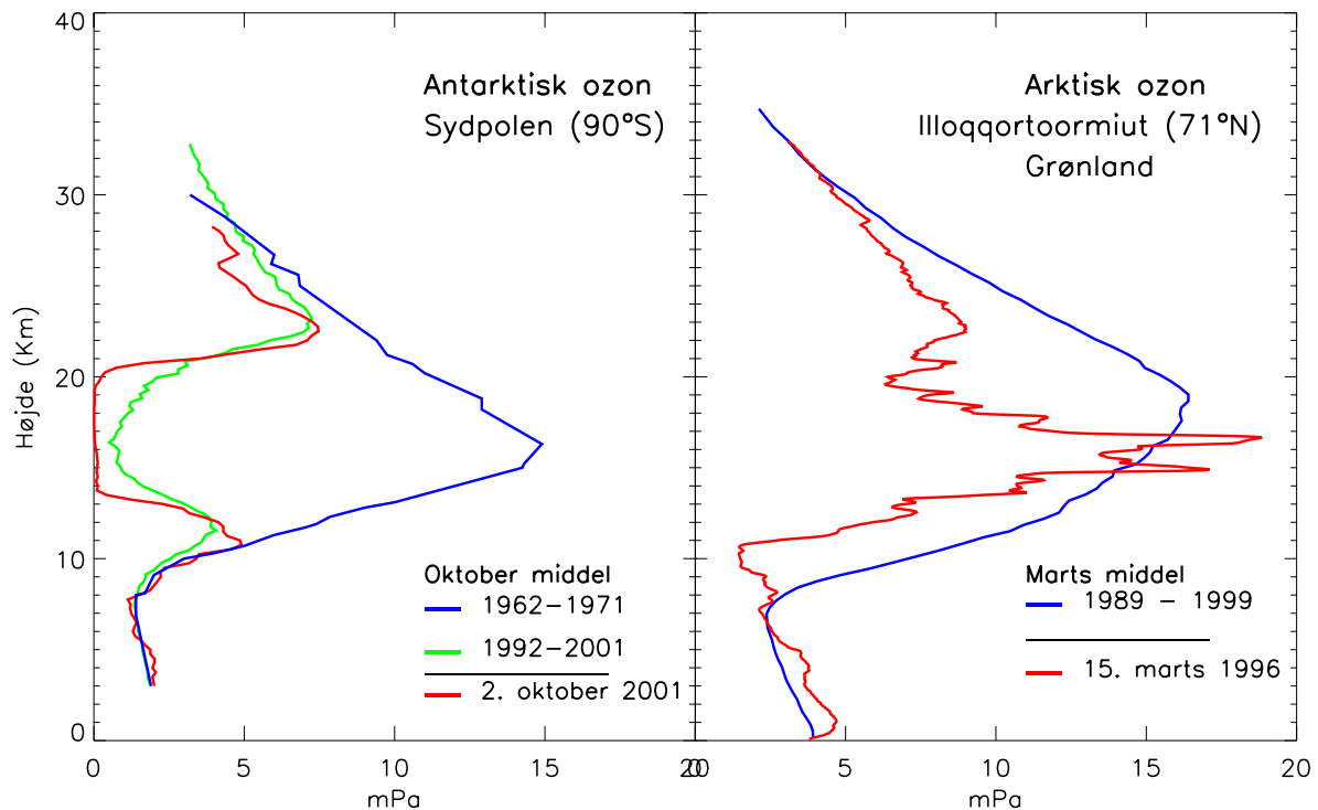
Figur 26. Højdeprofil af ozonnedbrydningen over Antarktis (til venstre) og Arktis (til højre). (WMO Assessment, 2002)
