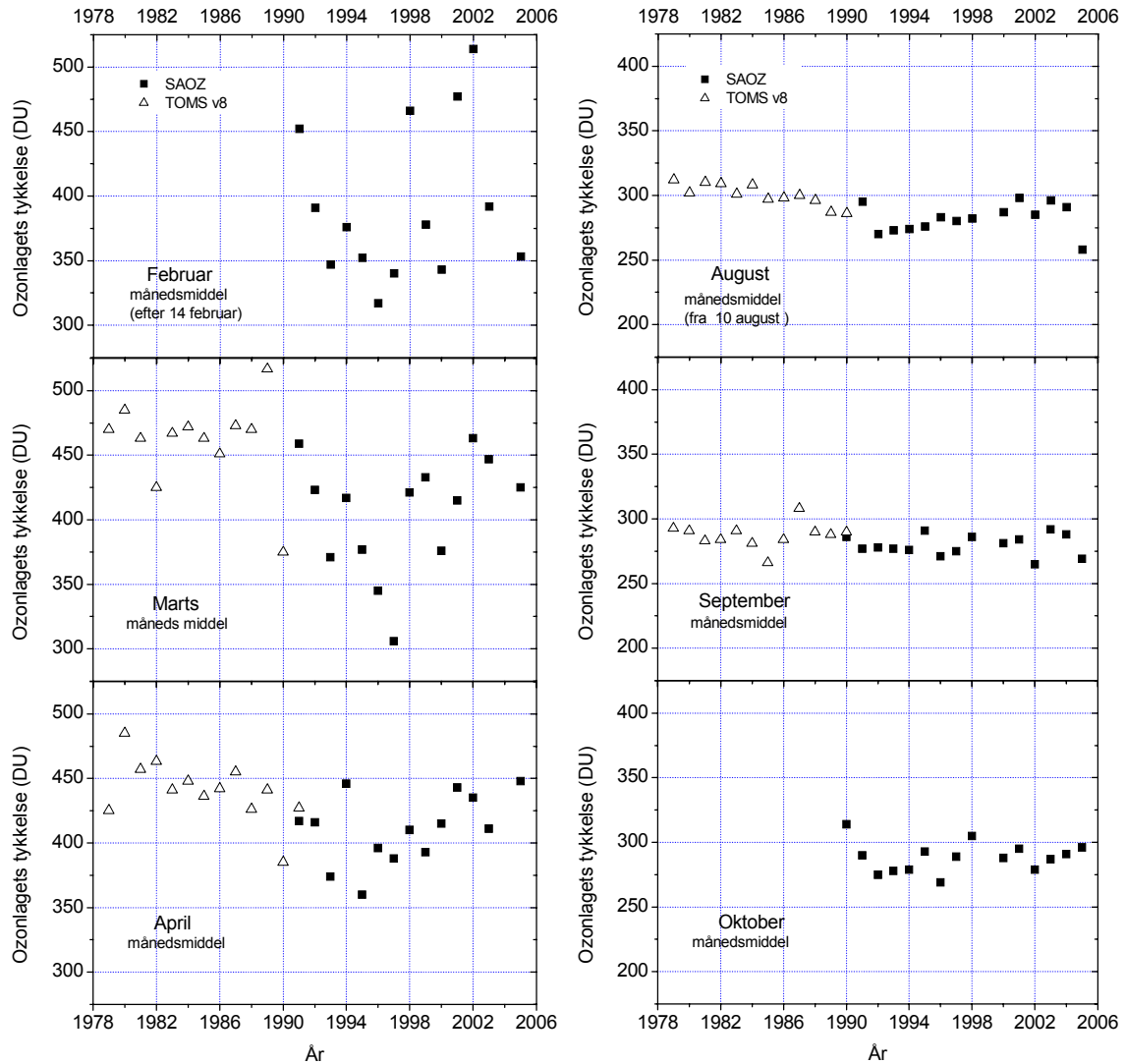
Figur 15. Månedsmidler af ozonlagets tykkelse over Pituffik. Data fra før september 1990 (trekanter) er målinger med NASAs TOMS-instrument. Data fra og med september 1990 (firkanter) er målinger med DMI's SAOZ-instrument.
