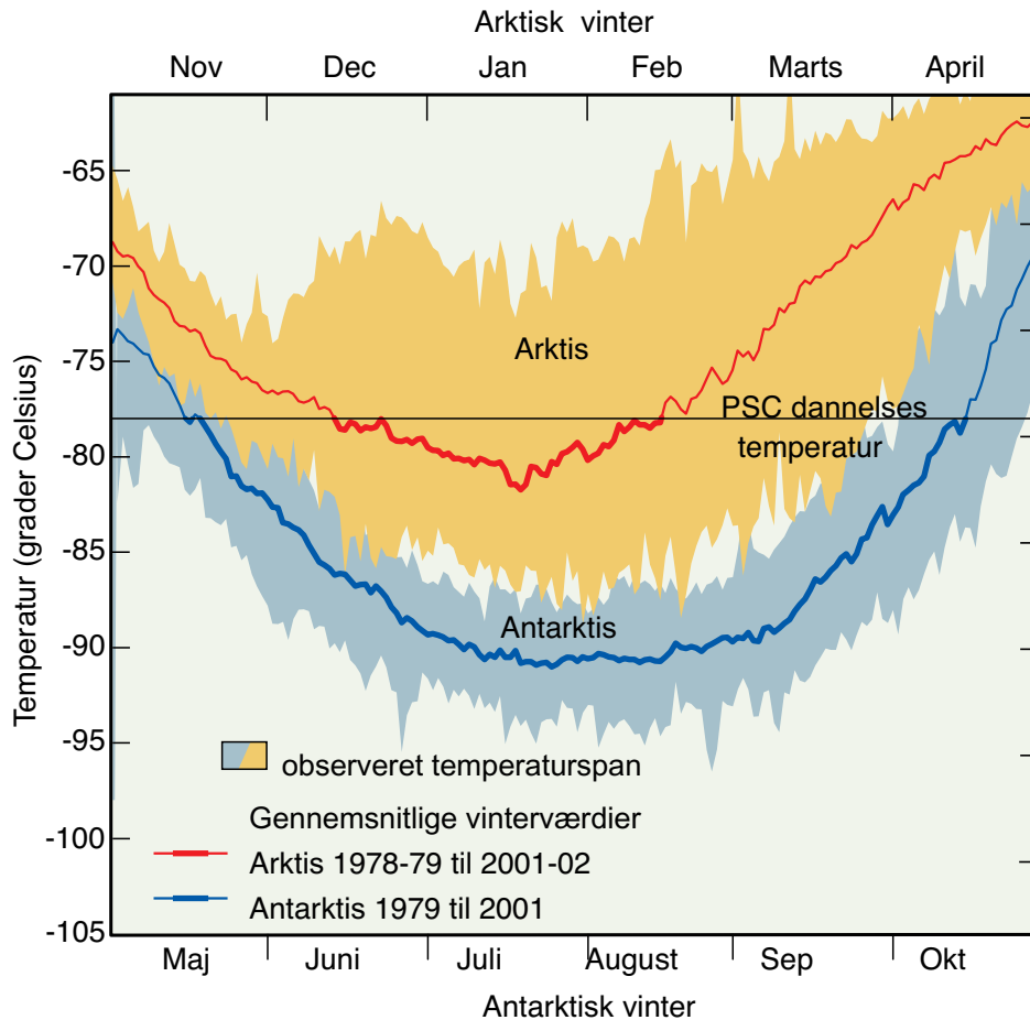
Figur 27. Minimumstemperaturer i Arktis og Antarktis. Den sorte linie angiver temperaturen, hvorunder PSC'er kan dannes. Den røde linie angiver gennemsnittet af minimumstemperaturen i Arktis gennem vintrene fra 1978-1979 til 2001-2002, mens det gule areal angiver hele det interval, inden for hvilket minimumstemperaturen svinger. Tilsvarende angiver den blå linie gennemsnittet af minimum temperaturen i Antarktis gennem vintrene 1979-2001, og det blå areal hele det interval, inden for hvilket minimumstemperaturen svinger. (WMO Assessment, 2002).
