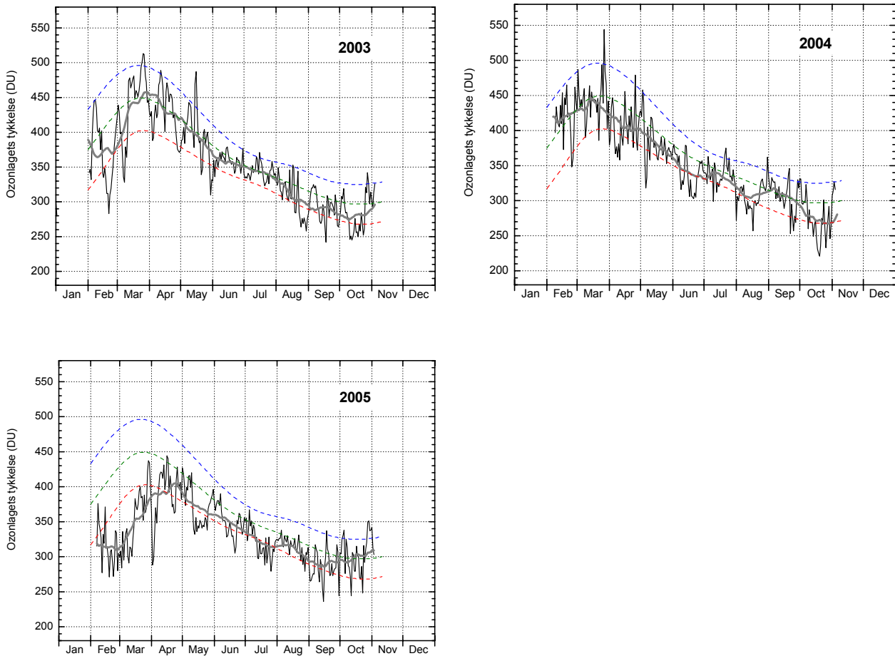
Figur 14. Ozonlagets tykkelse over Kangerlussuaq 2003-2005. Daglige målinger (tynd, sort linie) er DMI's målinger i Kangerlussuaq. Den grønne stiplede linie angiver middelværdien af daglige målinger i 10-års perioden 1979-1988, mens de blå og røde stiplede linier angiver henholdsvis middelværdien plus (blå) eller minus (rød) en standardafvigelse fra middelværdien. Det betyder, at ca. 2/3 af alle målinger i perioden 1979-1988 ligger mellem den blå og den røde linie. Den tykke grå linie er en 31-dages løbende middelværdi af de daglige målinger. En forholdsvis varm polar stratosfære i vintrene 2002-2003 og (især) 2003-2004 medfører ringe ozonnedbrydning.
