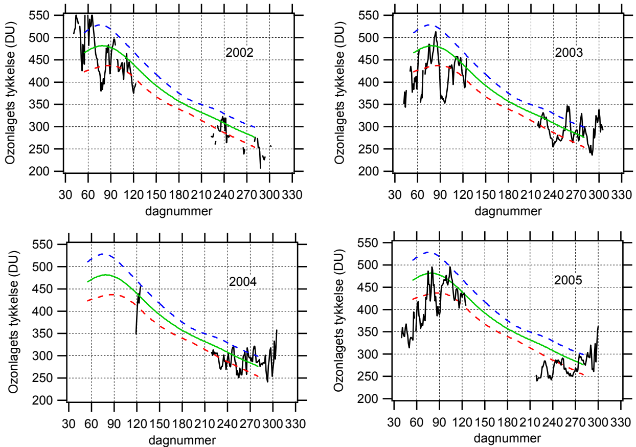
Figur 18. Ozonlagets tykkelse over Pituffik 2002-2005. Daglige målinger (sorte prikker) er DMI's målinger med SAOZ-spektrometeret. Den grønne linie angiver middelværdien af daglige målinger i ti-års perioden 1979-1988 målt med TOMS-instrumentet ombord på Nimbus7-satellitten. De blå og røde stiplede linier angiver plus og minus en standard afvigelse fra middelværdien. Det betyder, at 2/3 af alle målinger i perioden 1979-1988 ligger mellem den blå og den røde linie.
