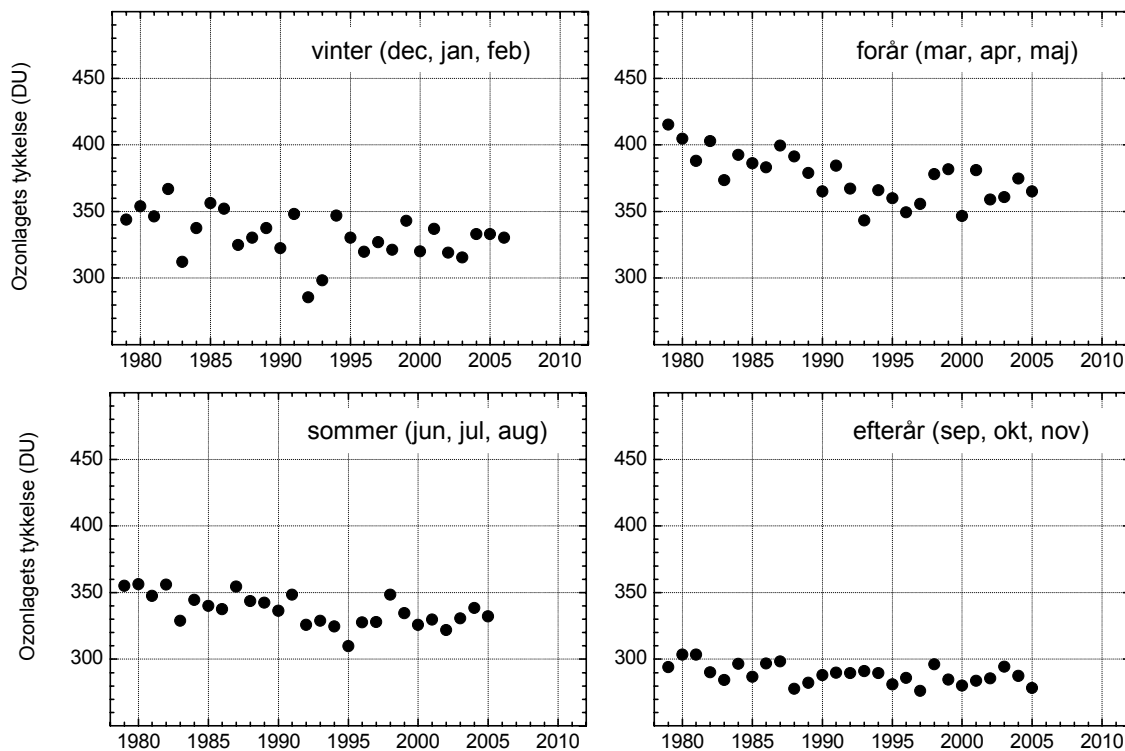
Figur 3. Ozonlagets sæsonmæssige middeltykkelse over Danmark for perioden 1979-2005. Data fra før 1993 er data fra NASA's TOMS-instrument på Nimbus7- satellitten. Data fra og med 1993 er DMI's målinger i København med et Brewer-instrument.
