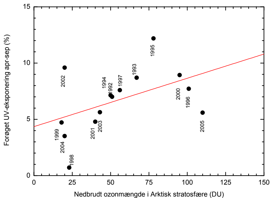
Figur 25. Beregnet sammenhæng mellem den ozonmængde der er nedbrudt i den arktiske stratosfære (14-24 km's højde) i perioden januar-marts og den forøgede UV-eksponering i Danmark i de efterfølgende 5 måneder (april-september). Som referenceniveau er anvendt middelværdien af ozonlagets tykkelse i 10-års perioden 1979-1988 (figur 4 og 5).
