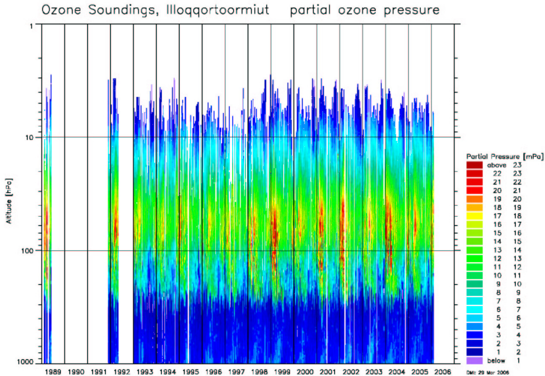
Figur 21. Oversigt over alle ozonsonderinger i Illoqqortoormiut. Figuren viser ozonens partialtryk som funktion af tid og trykhøjde. Se også figur A1 i appendiks 1.
