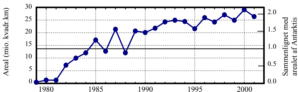
Figur 28. Det maksimale areal af det antarktiske ozonhul i perioden 1979-2001 (WMO Assessment, 2002).
