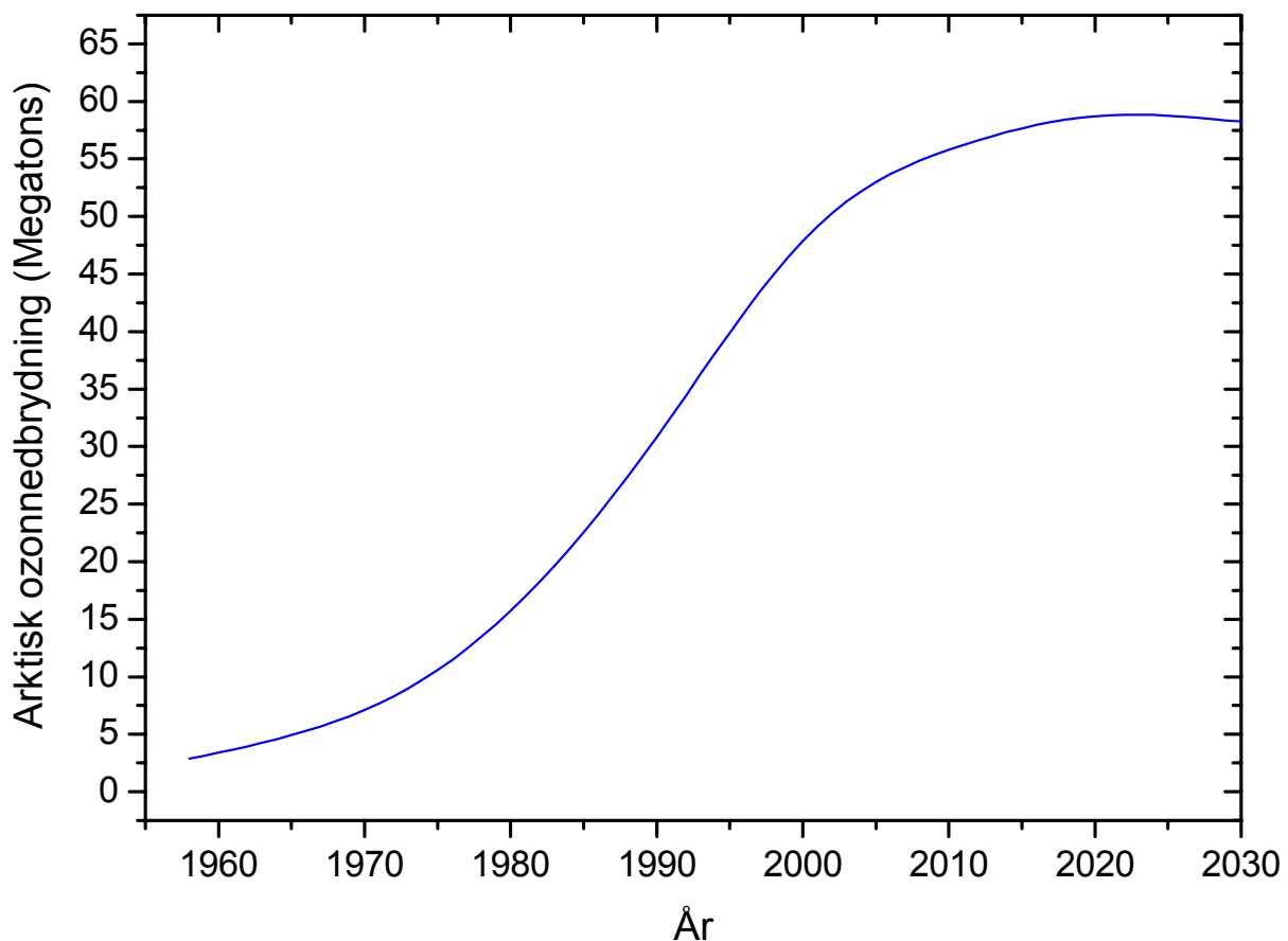
Figur 24: Forudsigelse af den arktiske ozonnedbrydning i de 20% koldeste vintre.
