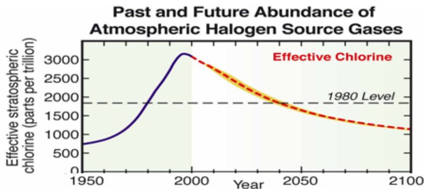
Figur 30. Mængden af ozonnedbrydende stoffer som funktion af tiden. Den fuldt optrukne del af linien baserer sig på målinger, mens den stiplede del af linien viser den forventede udvikling, hvis Montreal-protokollen med tilføjelser overholdes. Figuren er fra WMO (2003).
