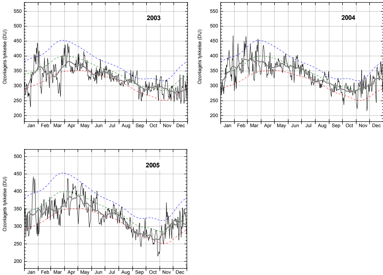
Figur 8. Ozonlagets tykkelse over Danmark 2003-2005. Daglige målinger (tynd, sort linie) er DMI's målinger i København. Den grønne stiplede linie angiver middelværdien af daglige målinger i 10-års perioden 1979-1988, mens de blå og røde stiplede linier angiver henholdsvis middelværdien plus (blå) eller minus (rød) en standardafvigelse fra middelværdien. Det betyder, at ca. 2/3 af alle målinger i perioden 1979-1988 ligger mellem den blå og den røde linie. Den tykke grå linie er en 31-dages løbende middelværdi af de daglige målinger. En forholdsvis varm polar stratosfære i vintrene 2002-2003 og (især) 2003-2004 med deraf følgende ringe ozonnedbrydning sætter sine spor i de følgende forår og somre med forholdsvis normalt ozonlag.
