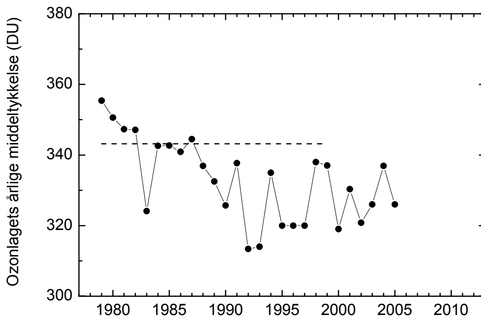
Figur 2. Ozonlagets årlige middeltykkelse over Danmark for perioden 1979-2005. Den gennemsnitlige udtynding af ozonlaget over perioden er 0,3% pr. år. Den gennemsnitlige årlige middelværdi for 10-års perioden 1979-1988 er 344 DU, vist med den stiplede linie. Betragtes alene de sidste 10 års data ses ingen tendens. Data fra før 1993 er data fra NASA's TOMS instrument på Nimbus7-satellitten. Data fra og med 1993 er DMI's målinger i København med et Brewer-instrument.
