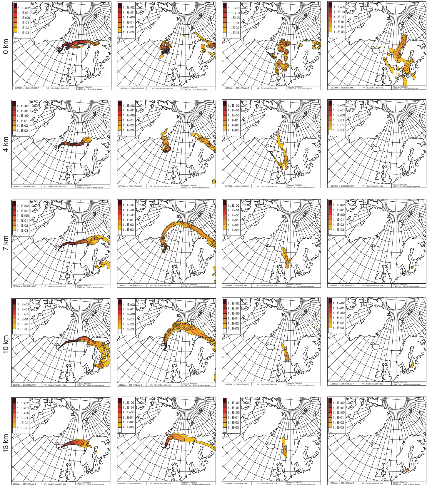
Koncentration i arbitrære enheder af vulkansk aske i højderne 0, 4, 7, 10 og 13 km over overfladen 0 UTC d. 3., 4., 5. og 6. november 2004. Beregningen er foretaget for den del af asken, som svarer til partikler af størrelse mindre end nogle få \mu\text{m} .
