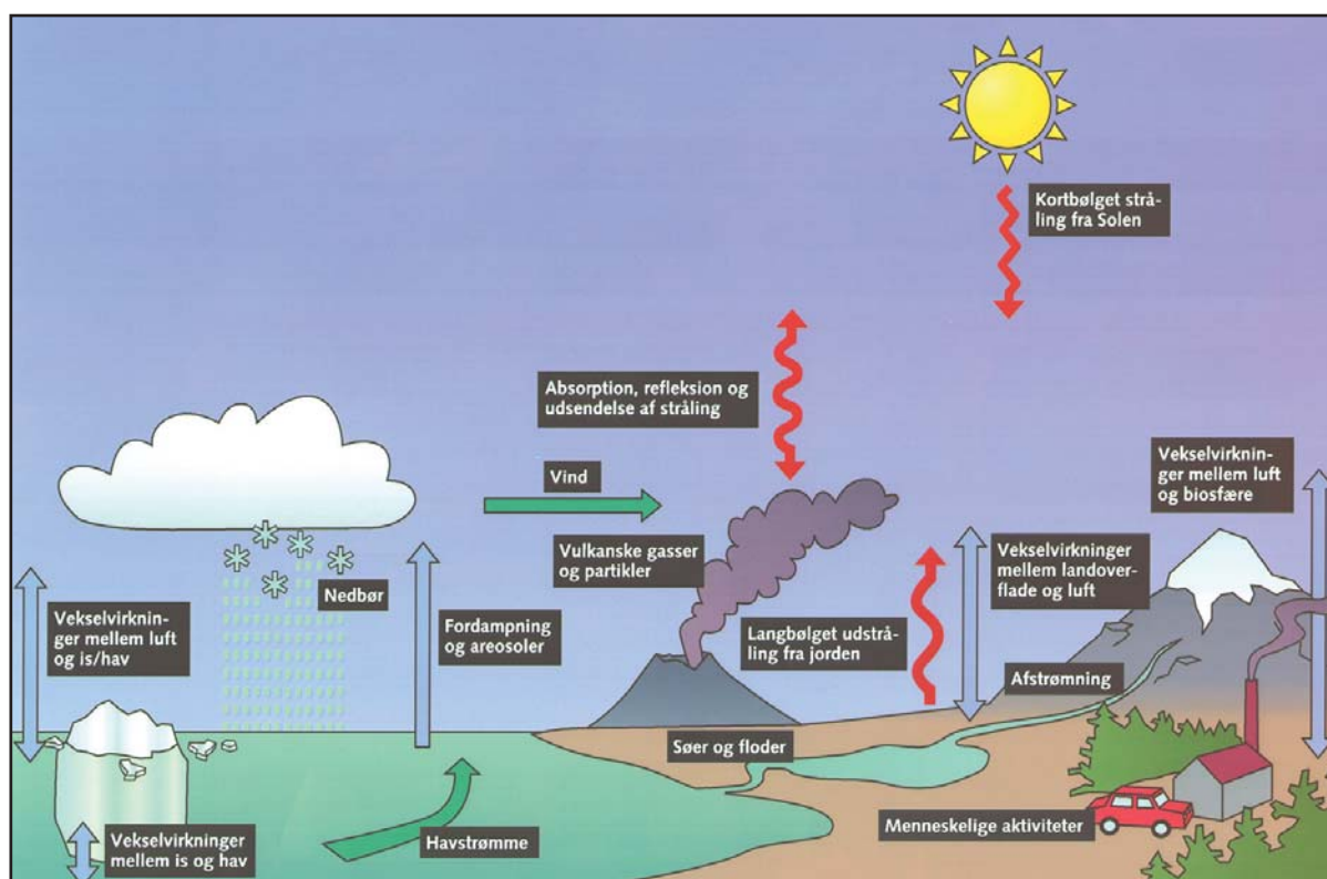
Klimasystemet og de processer, der beskrives i koblete atmosfære-ocean-klimamodeller. (Grafik: DMI)
