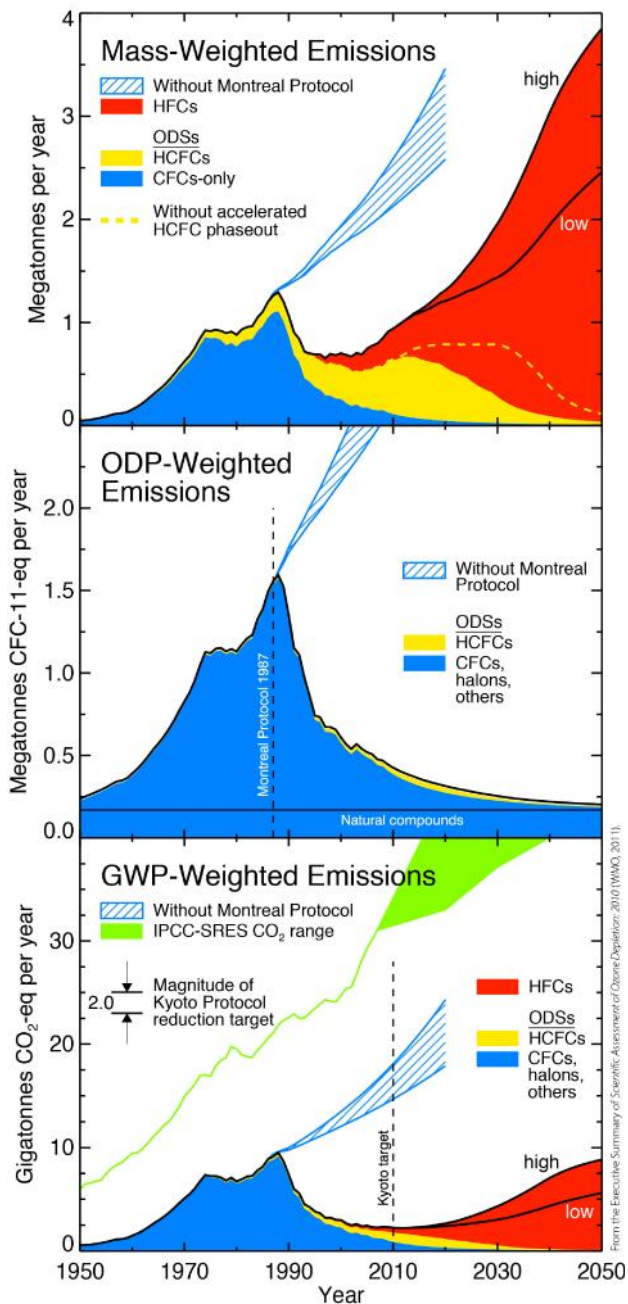
Figur C1 (fra WMO, 2011).
