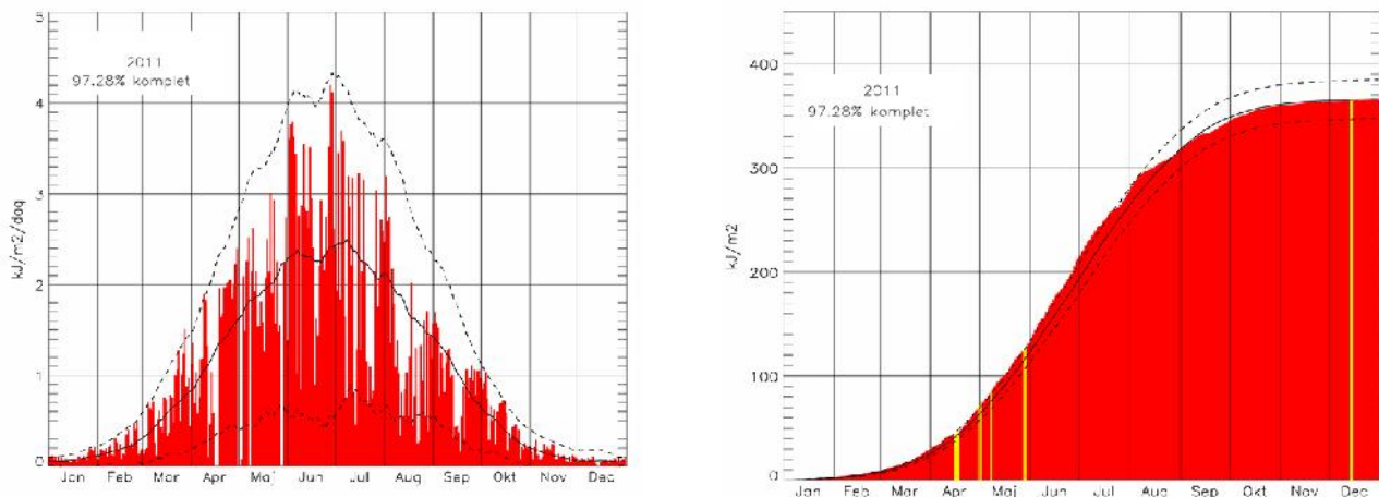
Figur 15 . (Venstre panel) Den dagligt målte totale dosis af hudskadelig UV stråling i 2011 i København i kJ/m 2 /dag. Fuldt optrukken kurve er den tilsvarende middel-dosis for 2000-2010. Øvre og nedre punkterede kurver viser hhv. +2 og -2 standardafvigelser. (Højre panel) Den totale dosis i løbet af året af hudskadelig UV stråling i 2011 i København i kJ/m 2 . Fuldt optrukken kurve er den tilsvarende middel-dosis for 2000-2010. Øvre og nedre punkterede kurver viser hhv. +2 og -2 standardafvigelser.
