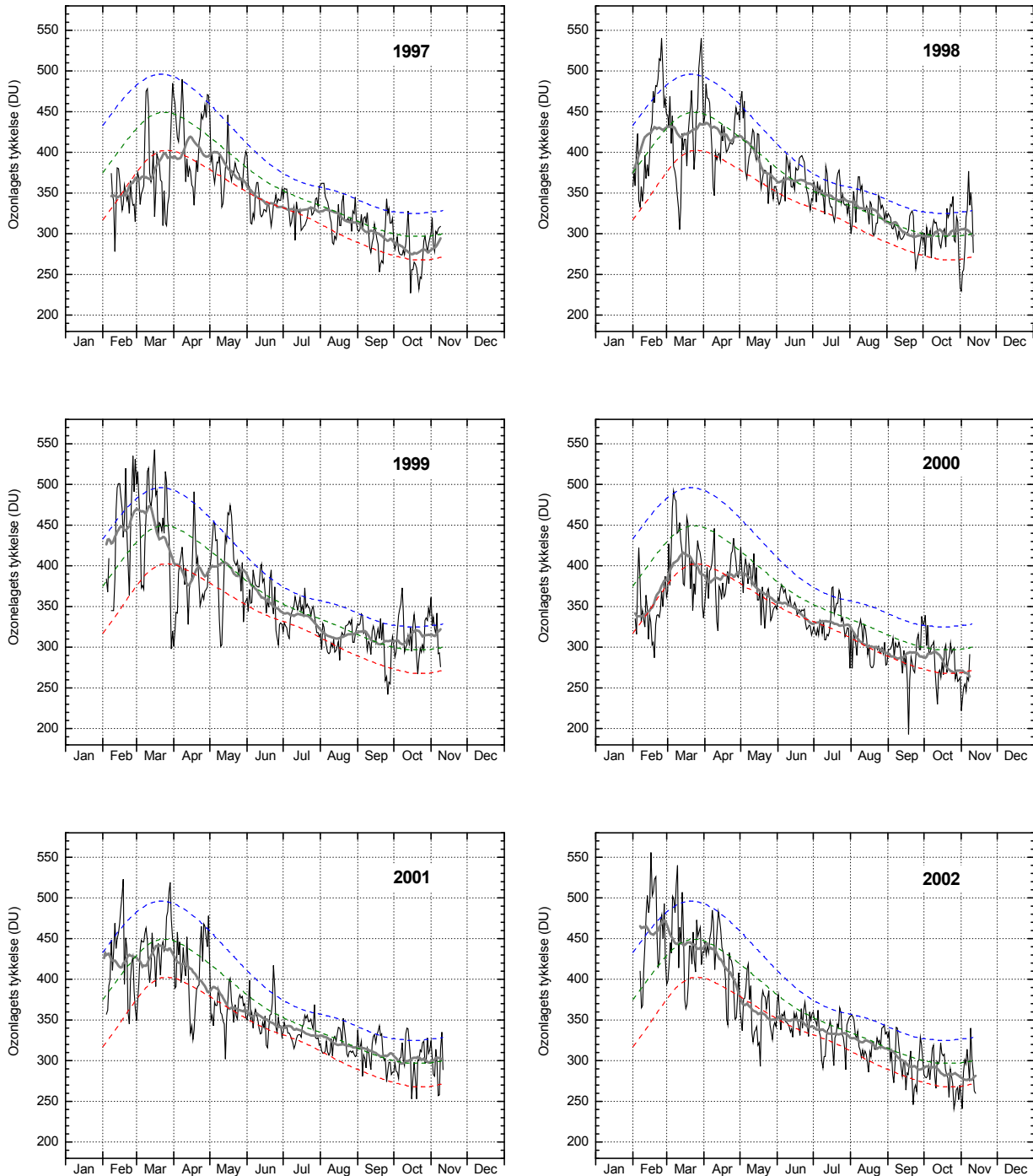
Figur A10. Ozonlagets tykkelse over Kangerlussuaq 1997-2002. Daglige målinger (tynd, sort linje) er DMI's målinger i Kangerlussuaq. Den grønne stiplede linje angiver middelværdien af daglige målinger i 10-års perioden 1979-1988, mens de blå og røde stiplede linjer angiver henholdsvis middelværdien plus (blå) eller minus (rød) en standardafvigelse fra middelværdien. Det betyder, at ca. 2/3 af alle målinger i perioden 1979-1988 ligger mellem den blå og den røde linje. Den tykke grå linje er en 31-dages løbende middelværdi af de daglige målinger. Forholdsvis stor ozonnedbrydning ses i den polare stratosfære i vinteren 1999-2000, mens en forholdsvis varm polar stratosfære i vintrene 1997-1998, 1998-1999, 2000-2001 og 2001-2002 medfører ringe ozonnedbrydning.
