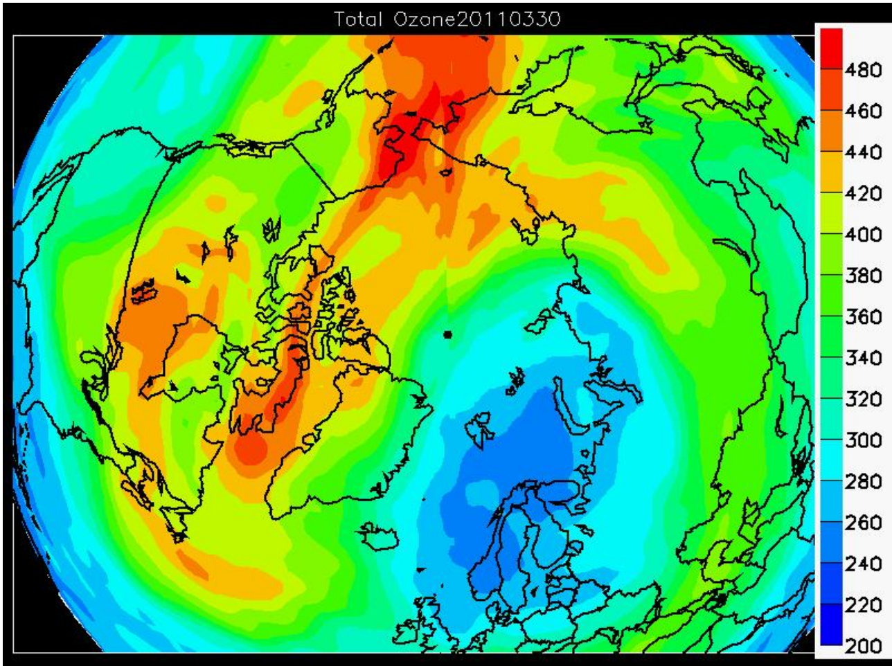
Figur 11. Ozonlagets tykkelse (DU) over den nordlige halvkugle 30. marts 2011, observeret fra Gome-2 instrument ombord på Eumetsat's MetOp satellit. Vorticet er drejet ind over Skandinavien, og inden for vorticet måles de lave tykkelser af ozonlaget ned til omkring 250 DU.
