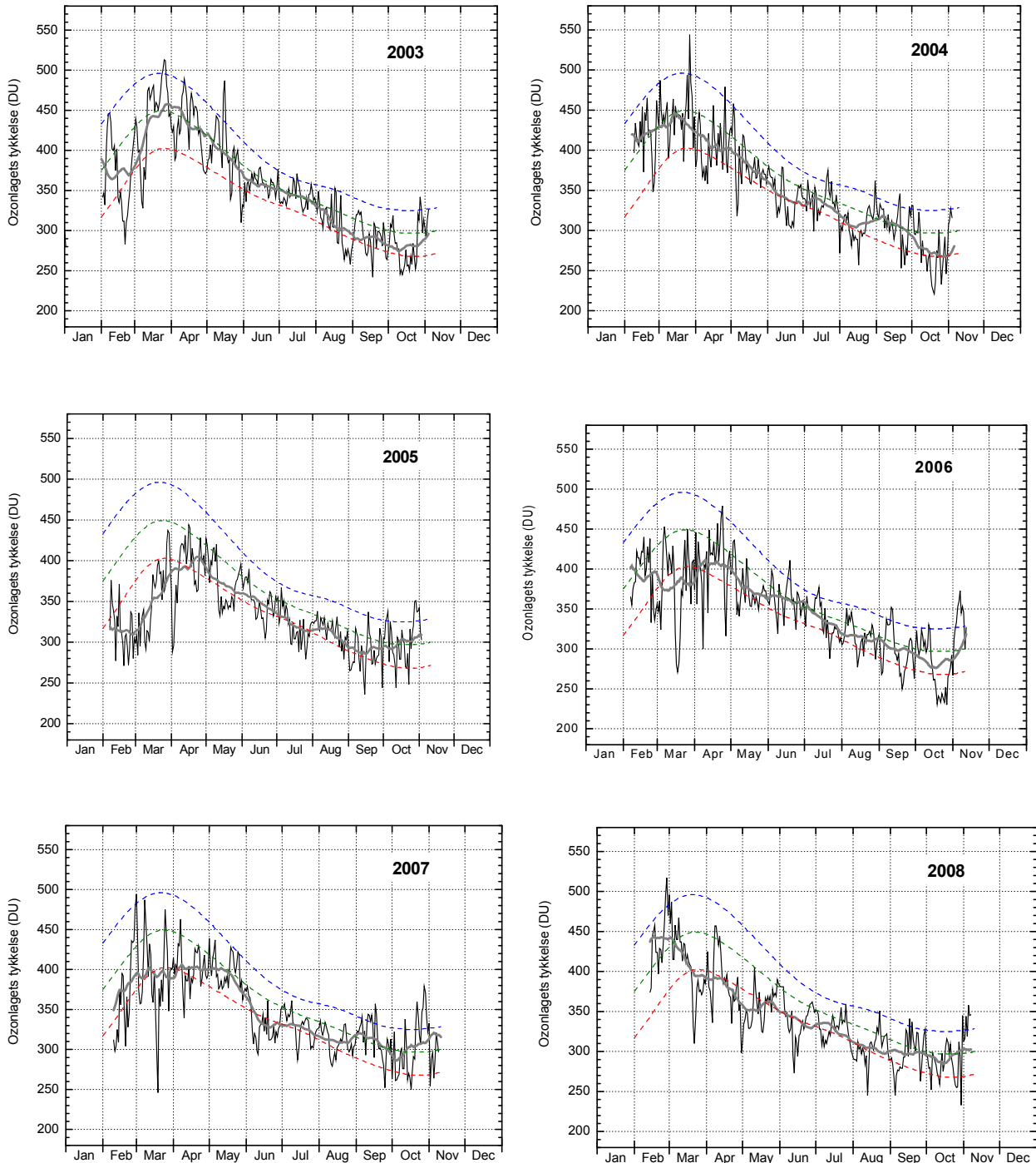
Figur A11. Ozonlagets tykkelse over Kangerlussuaq 2003-2008. Daglige målinger (tynd, sort linje) er DMI's målinger i Kangerlussuaq. Den grønne stiplede linje angiver middelværdien af daglige målinger i 10-års perioden 1979-1988, mens de blå og røde stiplede linjer angiver henholdsvis middelværdien plus (blå) eller minus (rød) en standardafvigelse fra middelværdien. Det betyder, at ca. 2/3 af alle målinger i perioden 1979-1988 ligger mellem den blå og den røde linje. Den tykke grå linje er en 31-dages løbende middelværdi af de daglige målinger. En forholdsvis varm polar stratosfære i vintrene 2002-2003 og (især) 2003-2004 medfører ringe ozonnedbrydning.
