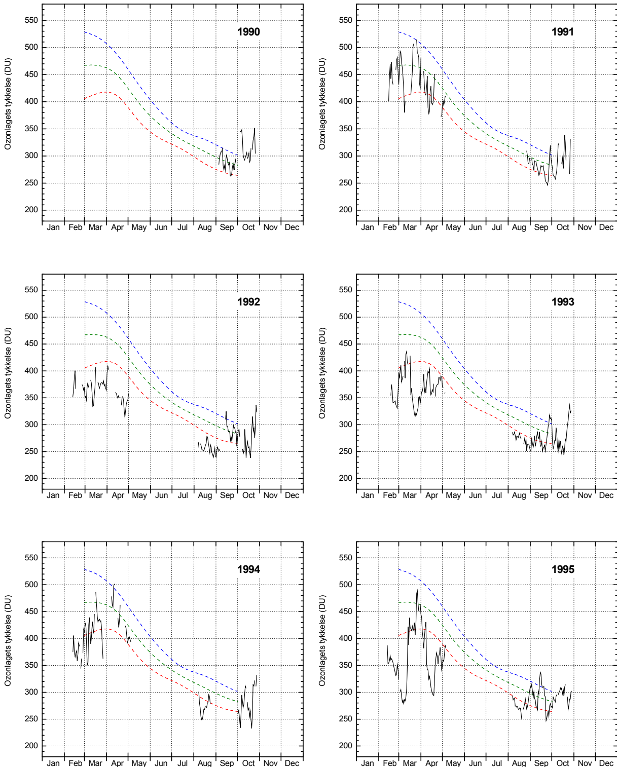
Figur A13. Ozonlagets tykkelse over Pituffik 1990-1995. Daglige målinger med SAOZ-spektrometeret. Den grønne linje angiver middelværdien af daglige målinger i ti-års perioden 1979-1988 målt med TOMS-instrumentet ombord på Nimbus7-satellitten. De blå og røde stiplede linjer angiver plus og minus en standardafvigelse fra middelværdien. Det betyder, at 2/3 af alle målinger i perioden 1979-1988 ligger mellem den blå og den røde linje.
