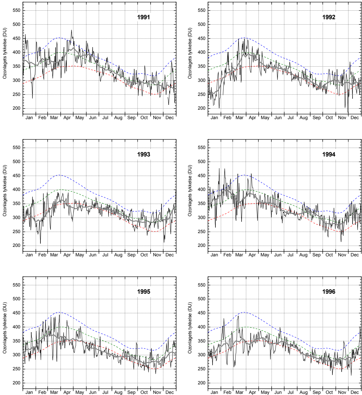
Figur A3. Ozonlagets tykkelse over Danmark 1991-1996. Daglige målinger (tynd, sort linje) frem til maj 1992 er fra NASA's TOMS-instrument på Nimbus7-satellitten, og fra og med juni 1992 DMI's daglige målinger i København. Den grønne stiplede linje angiver middelværdien af daglige målinger i 10-års perioden 1979-1988, mens de blå og røde stiplede linjer angiver henholdsvis middelværdien plus (blå) eller minus (rød) en standardafvigelse fra middelværdien. Det betyder, at ca. 2/3 af alle målinger i perioden 1979-1988 ligger mellem den blå og den røde linje. Den tykke grå linje er en 31-dages løbende middelværdi af de daglige målinger. Et kraftigt vulkanudbrud i juni 1991 (Mt. Pinatubo, Filippinerne) påvirker ozonlaget i 1992 og 1993. Forholdsvis stor ozonnedbrydning i den polare stratosfære i vintrene 1991-1992, 1992-1993, 1994-1995 og 1995-1996 sætter sine spor med forholdsvis tyndt ozonlag gennem de efterfølgende somre. I Danmark var sommeren 1995 desuden præget af langvarigt højtryk, hvilket også bidrog til et tyndt ozonlag.
