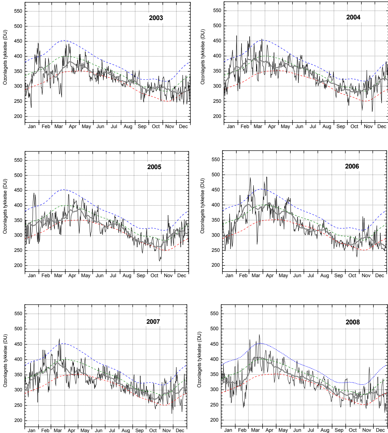
Figur A5. Ozonlagets tykkelse over Danmark 2003-2008. Daglige målinger (tynd, sort linje) er DMI's målinger i København. Den grønne stiplede linje angiver middelværdien af daglige målinger i 10-års perioden 1979-1988, mens de blå og røde stiplede linjer angiver henholdsvis middelværdien plus (blå) eller minus (rød) en standardafvigelse fra middelværdien. Det betyder, at ca. 2/3 af alle målinger i perioden 1979-1988 ligger mellem den blå og den røde linje. Den tykke grå linje er en 31-dages løbende middelværdi af de daglige målinger. En forholdsvis varm polar stratosfære i vintrene 2002-2003 og (især) 2003-2004 med deraf følgende ringe ozonnedbrydning sætter sine spor i de følgende forår og somre med forholdsvis normalt ozonlag.
