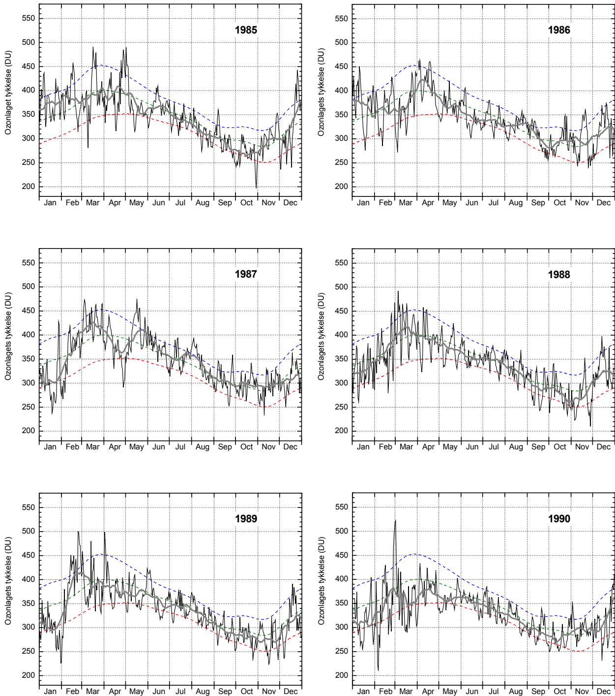
Figur A2. Ozonlagets tykkelse over Danmark 1985-1990. Daglige målinger (tynd, sort linje) er fra NASA's TOMS-instrument på Nimbus7-satellitten. Den grønne stiplede linje angiver middelværdien af daglige målinger i 10-års perioden 1979-1988, mens de blå og røde stiplede linjer angiver henholdsvis middelværdien plus (blå) eller minus (rød) en standardafvigelse fra middelværdien. Det betyder, at ca. 2/3 af alle målinger i perioden 1979-1988 ligger mellem den blå og den røde linje. Den tykke grå linje er en 31-dages løbende middelværdi af de daglige målinger.
