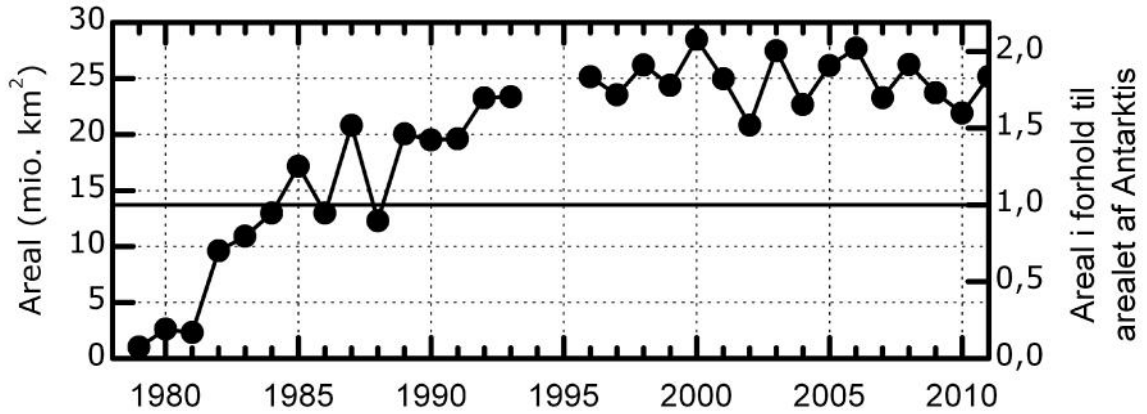
Figur 18. Det maksimale areal af det antarktiske ozonhul i perioden 1979-2011.
