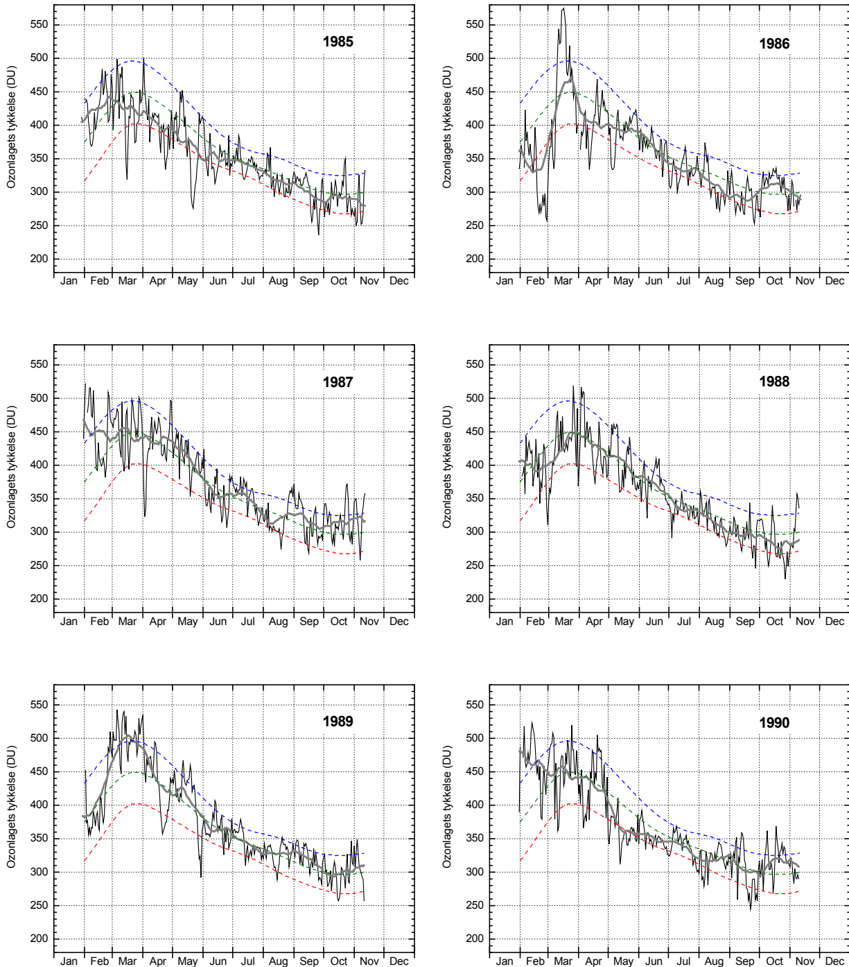
Figur A8. Ozonlagets tykkelse over Kangerlussuaq 1985-1990. Daglige målinger (tynd, sort linje) er fra NASA's TOMS instrument på Nimbus 7 satellitten. Den grønne stiplede linje angiver middelværdien af daglige målinger i 10-års perioden 1979-1988, mens de blå og røde stiplede linjer angiver henholdsvis middelværdien plus (blå) eller minus (rød) en standardafvigelse fra middelværdien. Det betyder, at ca. 2/3 af alle målinger i perioden 1979-1988 ligger mellem den blå og den røde linje. Den tykke grå linje er en 31-dages løbende middelværdi af de daglige målinger.
