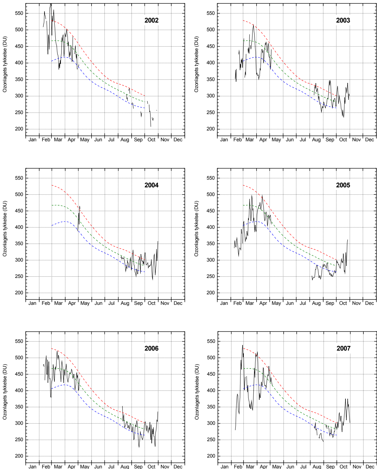
Figur A15. Ozonlagets tykkelse over Pituffik 2002-2007. Daglige målinger med SAOZ-spektrometeret. Den grønne linje angiver middelværdien af daglige målinger i ti-års perioden 1979-1988 målt med TOMS-instrumentet ombord på Nimbus7-satellitten. De blå og røde stiplede linjer angiver plus og minus en standard afvigelse fra middelværdien. Det betyder, at 2/3 af alle målinger i perioden 1979-1988 ligger mellem den blå og den røde linje.
