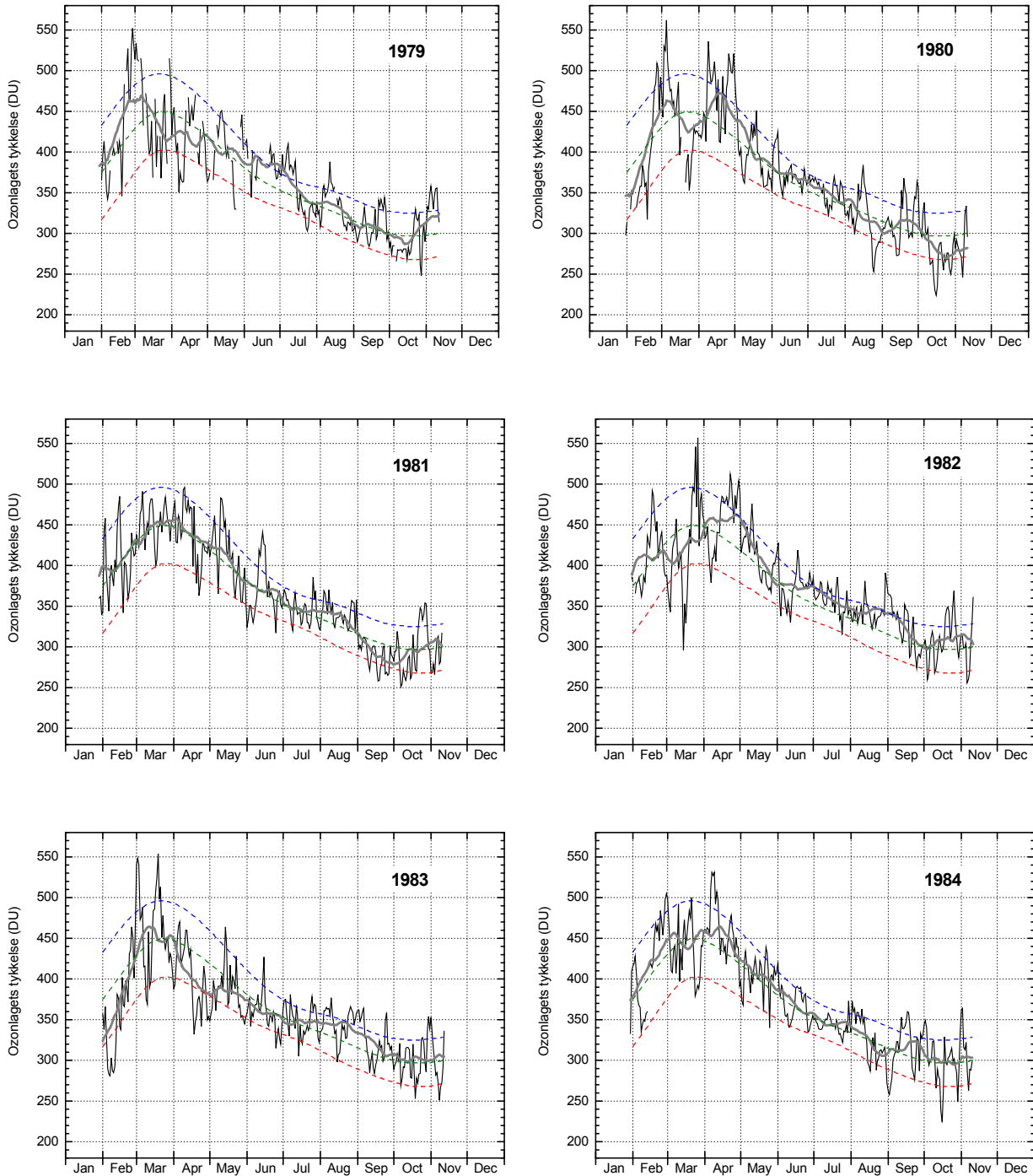
Figur A7. Ozonlagets tykkelse over Kangerlussuaq 1979-1984. Daglige målinger (tynd, sort linje) er fra NASA's TOMS instrument på Nimbus7-satellitten. Den grønne stiplede linje angiver middelværdien af daglige målinger i 10-års perioden 1979-1988, mens de blå og røde stiplede linjer angiver henholdsvis middelværdien plus (blå) eller minus (rød) en standardafvigelse fra middelværdien. Det betyder, at ca. 2/3 af alle målinger i perioden 1979-1988 ligger mellem den blå og den røde linje. Den tykke grå linje er en 31-dages løbende middelværdi af de daglige målinger.
