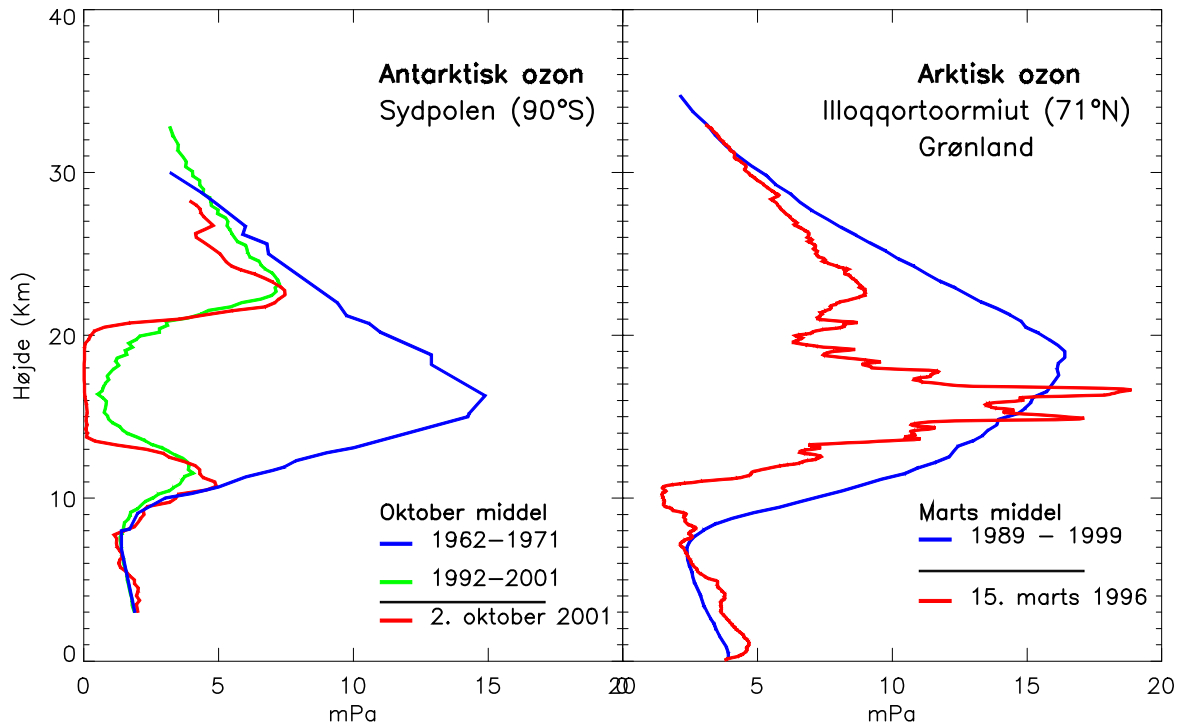
Figur 16. Højdeprofil af ozonnedbrydningen over Antarktis (til venstre) og Arktis (til højre). (WMO Assessment, 2002)
