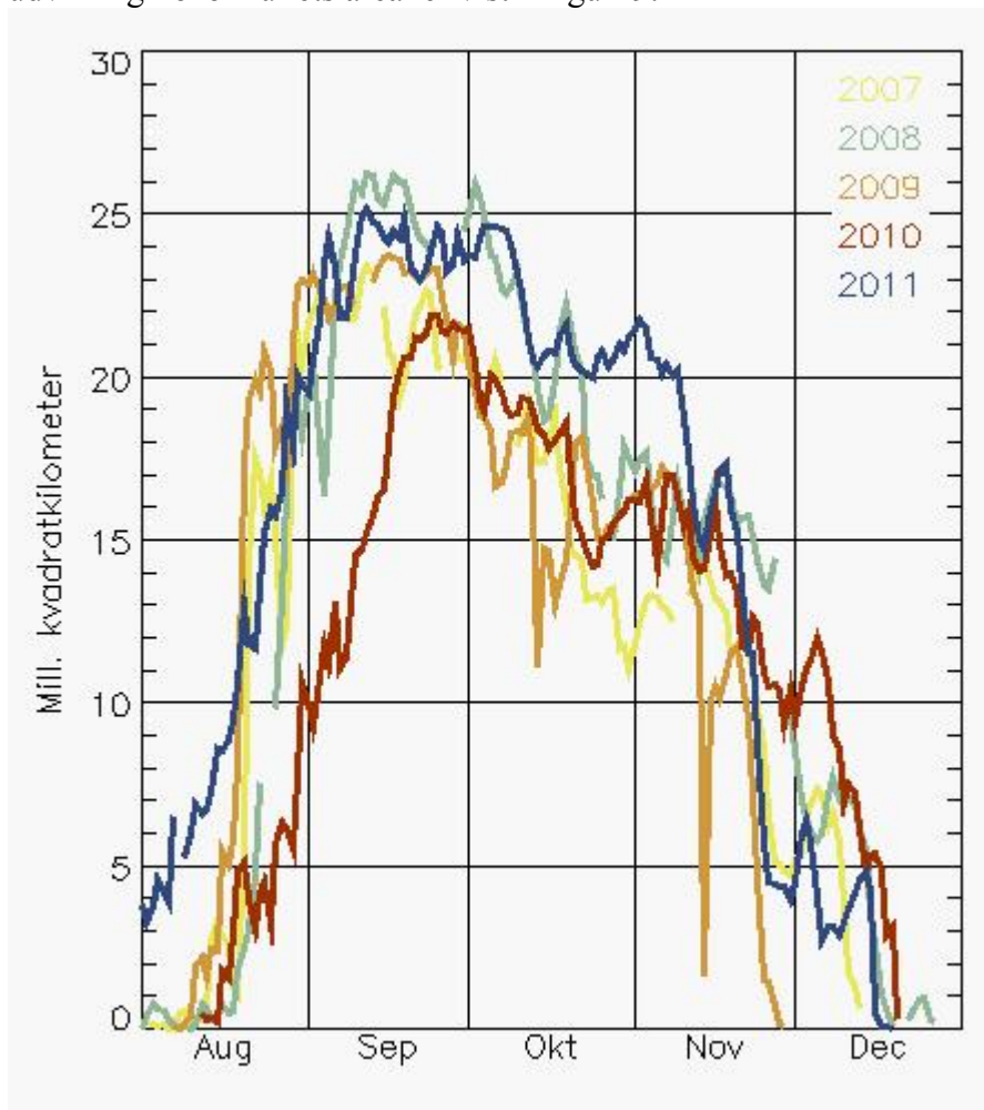
Figur 19. Udviklingen i det antarktiske ozonhuls areal de seneste 5 år.
