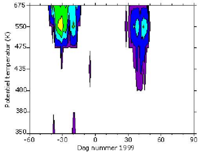
Figur A17b. Areal af den nordlige halvkugle dækket af PSC'ere i højdeinterval 350-675 K potentiel temperatur, svarende til ca. 14-26 km gennem vintrene 1999-2003.
