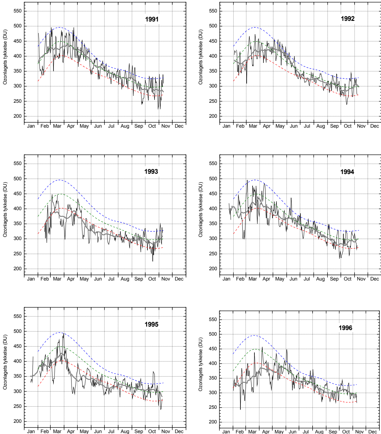
Figur A9. Ozonlagets tykkelse over Kangerlussuaq 1991-1996. Daglige målinger (tynd, sort linje) er DMI's målinger i Kangerlussuaq. Den grønne stiplede linje angiver middelværdien af daglige målinger i 10-års perioden 1979-1988, mens de blå og røde stiplede linjer angiver henholdsvis middelværdien plus (blå) eller minus (rød) en standardafvigelse fra middelværdien. Det betyder, at ca. 2/3 af alle målinger i perioden 1979-1988 ligger mellem den blå og den røde linje. Den tykke grå linje er en 31-dages løbende middelværdi af de daglige målinger. Virkningen af et kraftigt vulkanudbrud i juni 1991 (Mt. Pinatubo, Filippinerne) ses i 1992-1993. Forholdsvis stor ozonnedbrydning i den polare stratosfære i vintrene 1991-1992, 1992-1993, 1994-1995 og 1995-1996 sætter sine spor når den polare hvirvelvind er over Kangerlussuaq, hvilket tydeligt ses i februar, marts og april 1996.
