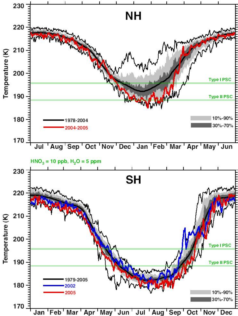
Figur 17. Årlig stratosfærisk temperatur cyklus og variabilitet i Arktis (NH) og Antarktis (SH). De grønne linjer angiver temperaturen, hvorunder PSC'er kan dannes. Den sorte kurve angiver middeltemperatur i perioden 1979-2004 (NH) og 1979-2005 (SH) med angivelse af rekordværdier (tynde sorte kurver). Den røde linje angiver udviklingen i Arktis (2004/2005) og Antarktis (2005) og 2002 (blå). Det grå areal angiver det interval, inden for hvilket procentdelen af observationerne falder. (WMO Assessment, 2007).
