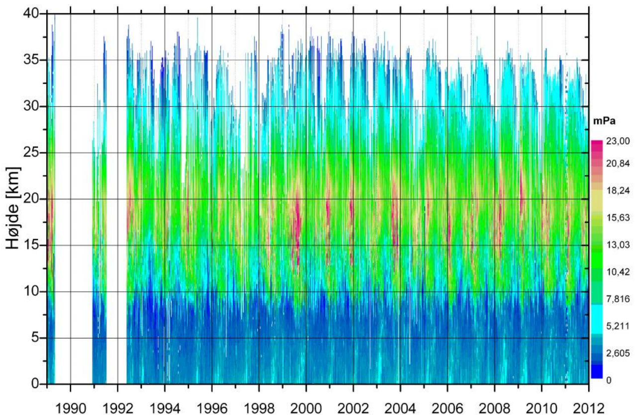
Figur 6. Oversigt over alle ozonsonderinger i Illoqqortoormiut. Figuren viser ozonens partialtryk som funktion af tid og højde. Se også figur B1 i appendiks B.
