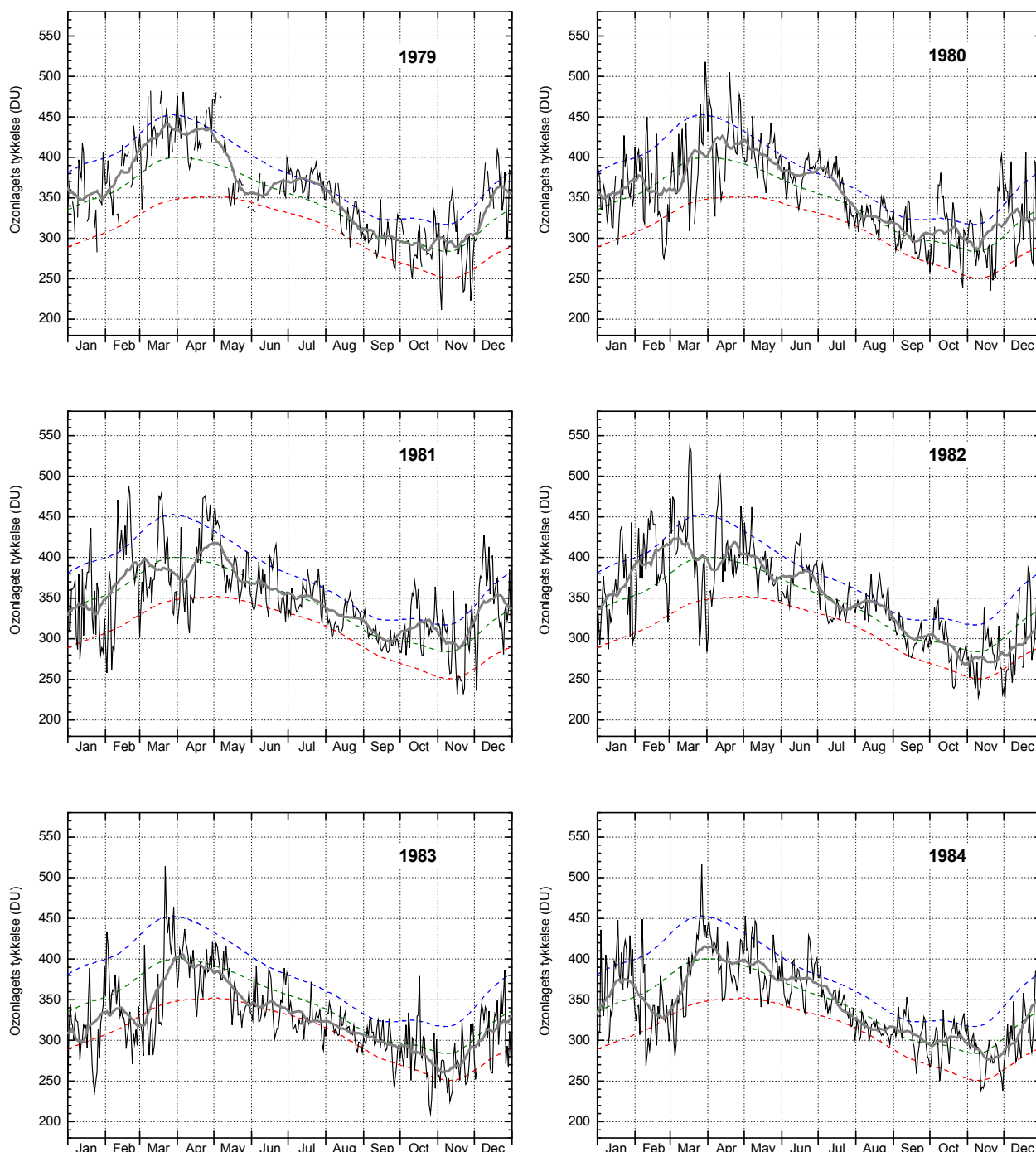
Figur A1. Ozonlagets tykkelse over Danmark 1979-1984. Daglige målinger (tynd, sort linje) er fra NASA's TOMS-instrument på Nimbus7-satellitten. Den grønne stiplede linje angiver middelværdien af daglige målinger i 10-års perioden 1979-1988, mens de blå og røde stiplede linjer angiver henholdsvis middelværdien plus (blå) eller minus (rød) en standardafvigelse fra middelværdien. Det betyder, at ca. 2/3 af alle målinger i perioden 1979-1988 ligger mellem den blå og den røde linje. Den tykke grå linje er en 31-dages løbende middelværdi af de daglige målinger. Nogle kraftige vulkanudbrud fandt sted mellem 28. marts og 4. april 1982 (El Chichon, Mexico). Sandsynligvis skyldes det gennemsnitligt noget tynde ozonlag i 1983 dette vulkanudbrud.
