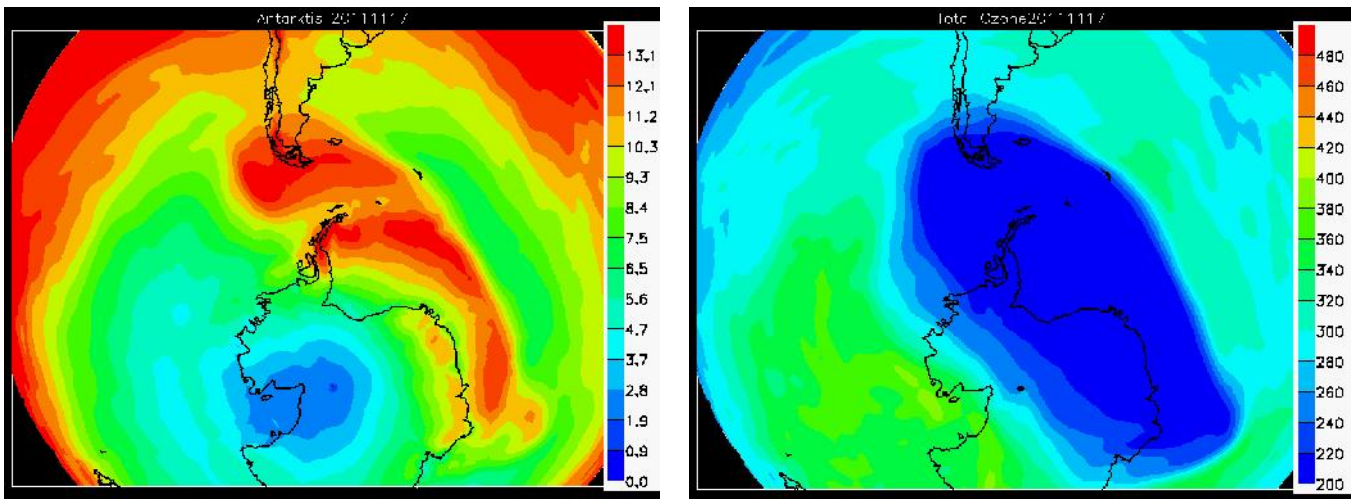
Figur 20. Beregnede UV-indices over det sydlige Amerika 17. november 2011 (venstre panel, UV-index) i forbindelse med det antarktiske ozonhul (højre panel, DU).
