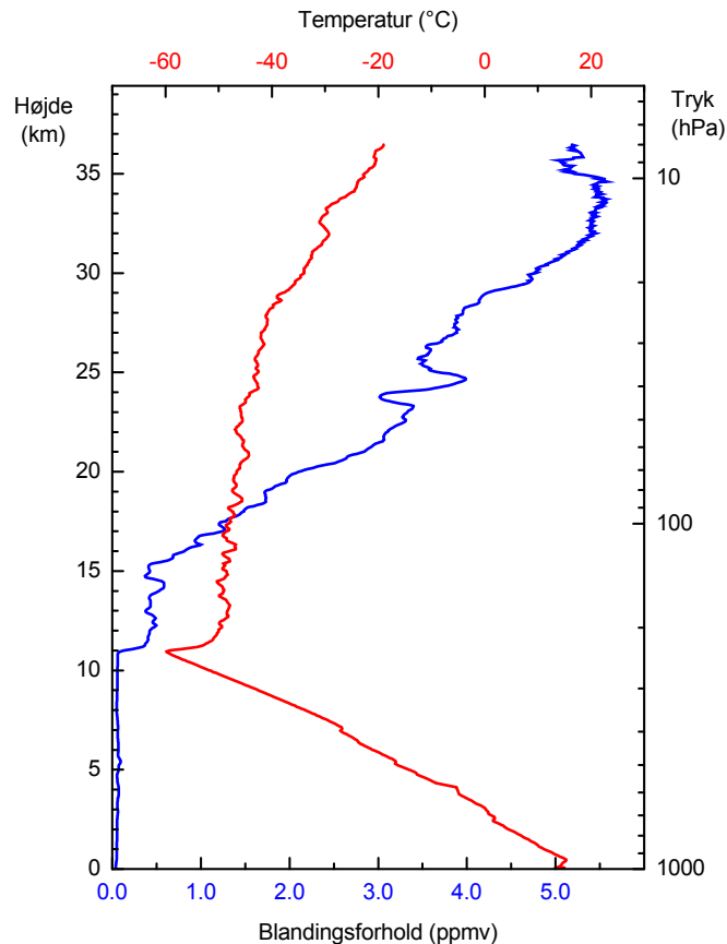
Figur B2. Ozon- og temperaturprofil fra Illoqqortoormiut (Scoresbysund), Grønland, den 13. juli 1994 målt med en ozonsonde. Den samme profil som vist i figur A1, blot med en anden enhed for ozonkoncentrationen. Blandingsforholdet angiver, hvor mange ozonmolekyler der findes for hver million molekyler i den omgivende luft. Skala for ozon er nederst, for temperatur øverst.
