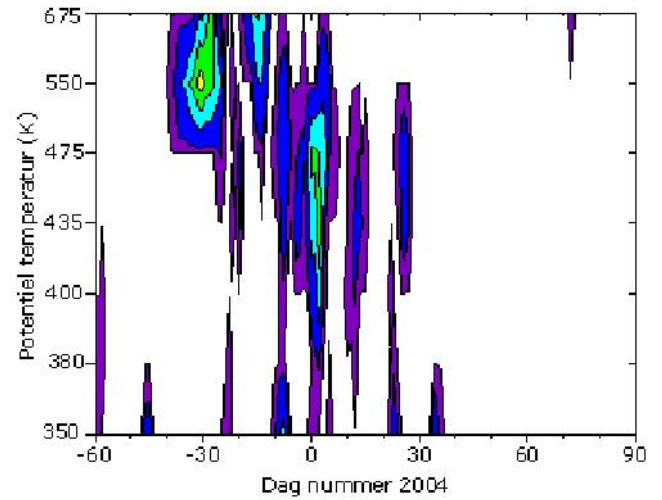
Figur A17c. Areal af den nordlige halvkugle dækket af PSC'ere i højdeinterval 350-675 K potentiel temperatur, svarende til ca. 14-26 km gennem vintrene 2004-2008.
