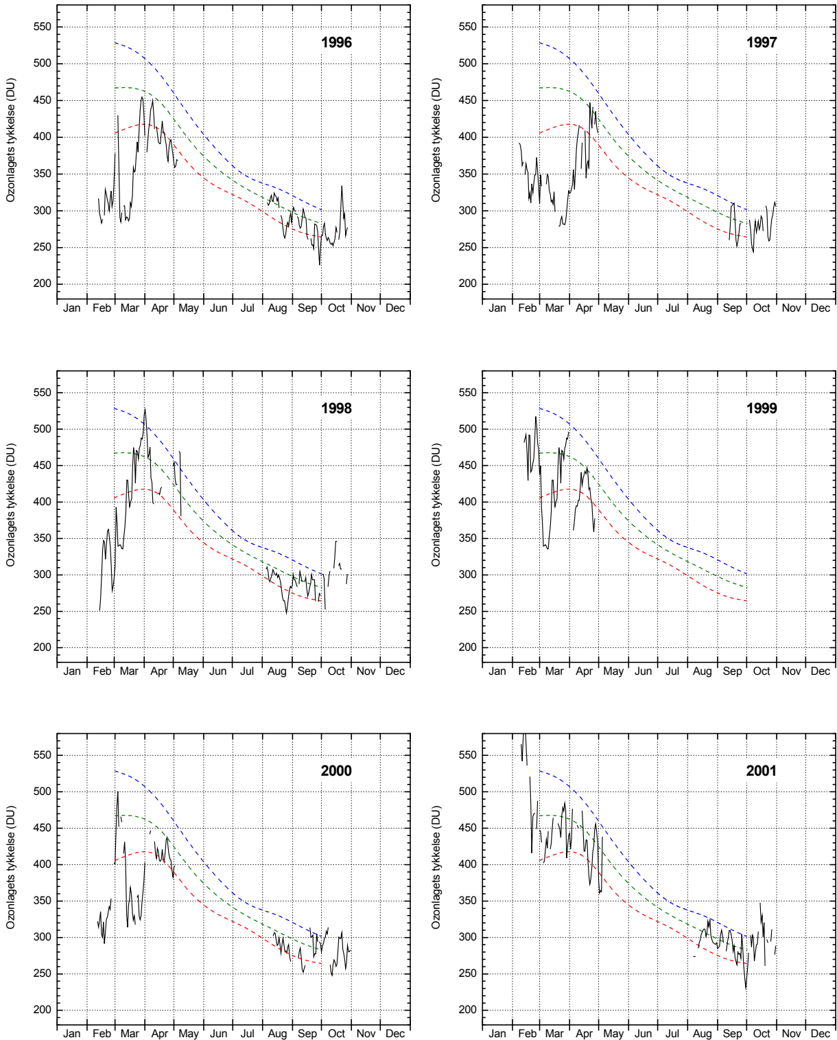
Figur A14. Ozonlagets tykkelse over Pituffik 1996-2001. Daglige målinger med SAOZ-spektrometeret. Den grønne linje angiver middelværdien af daglige målinger i ti-års perioden 1979-1988 målt med TOMS-instrumentet ombord på Nimbus7-satellitten. De blå og røde stiplede linjer angiver plus og minus en standardafvigelse fra middelværdien. Det betyder, at 2/3 af alle målinger i perioden 1979-1988 ligger mellem den blå og den røde linje.
