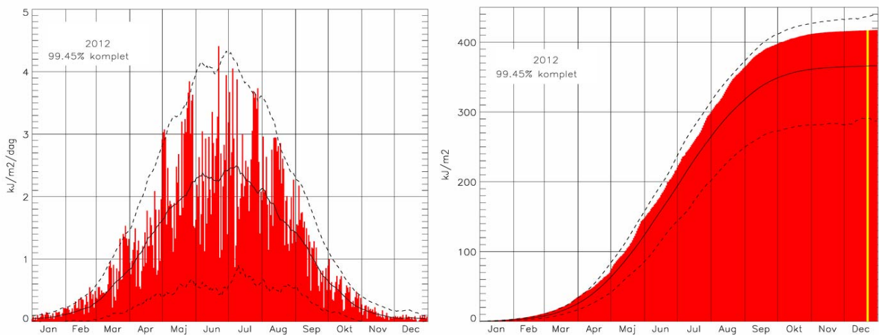
Figur 11 . (Venstre panel) Den dagligt målte totale dosis af hudskadelig UV stråling i 2012 i København i kJ/m 2 /dag. Fuldt optrukken kurve er den tilsvarende middel-dosis for 2000-2010. Øvre og nedre punkterede kurver viser hhv. +2 og -2 standardafvigelser. (Højre panel) Den totale dosis i løbet af året af hudskadelig UV stråling i 2012 i København i kJ/m 2 . Fuldt optrukken kurve er den tilsvarende middel-dosis for 2000-2010. Øvre og nedre punkterede kurver viser hhv. +2 og -2 standardafvigelser.
