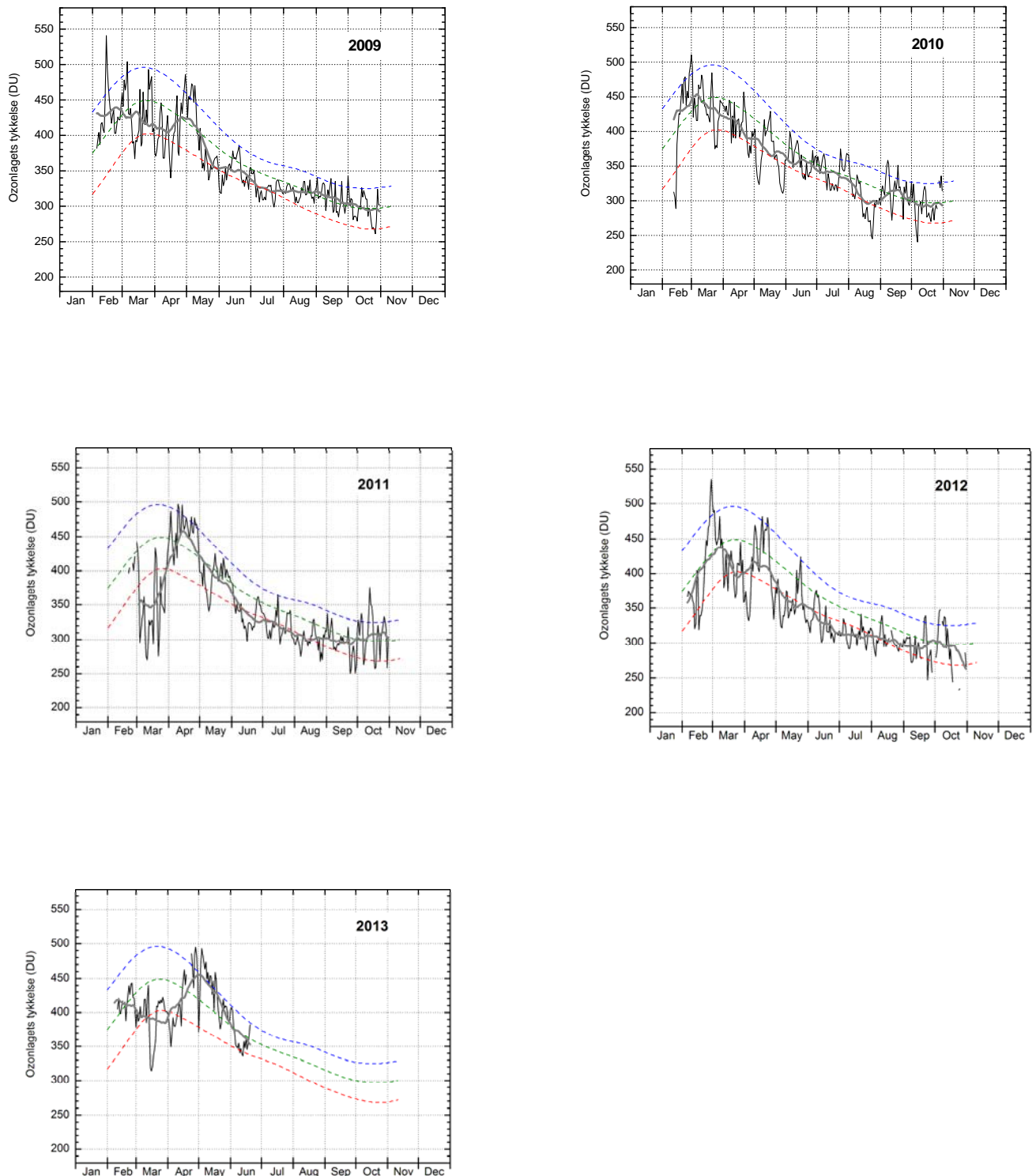
Figur A12. Ozonlagets tykkelse over Kangerlussuaq 2009-2013. Daglige målinger (tynd, sort linje) er DMI's målinger i Kangerlussuaq. Den grønne stiplede linje angiver middelværdien af daglige målinger i 10-års perioden 1979-1988, mens de blå og røde stiplede linjer angiver henholdsvis middelværdien plus (blå) eller minus (rød) en standardafvigelse fra middelværdien. Det betyder, at ca. 2/3 af alle målinger i perioden 1979-1988 ligger mellem den blå og den røde linje. Den tykke grå linje er en 31-dages løbende middelværdi af de daglige målinger.
