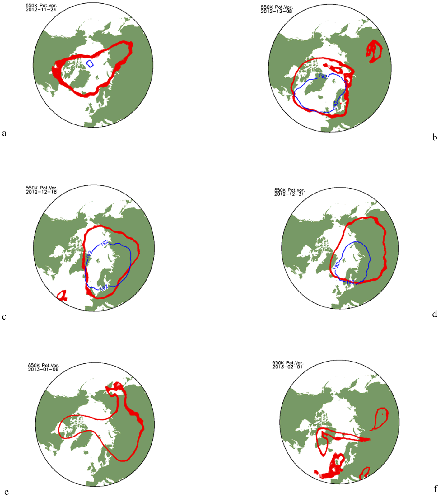
Figur 7. Røde konturlinjer viser grænsen for den polare vortex i 550 K potentieltemperaturshøjde, svarende til ca. 23 km, i perioden 24. november 2012 – 1. februar 2013. Blå konturlinjer viser isothermen for dannelse af type 1 polar-stratosfæriske skyer.
