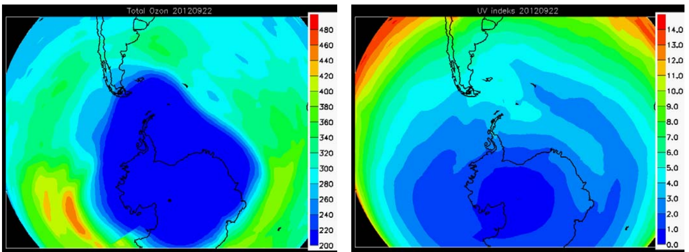
Figur 16. Beregnede UV-indices over det sydlige Amerika 22. september 2012 (højre panel) i forbindelse med det antarktiske ozonhul (venstre panel, DU).
