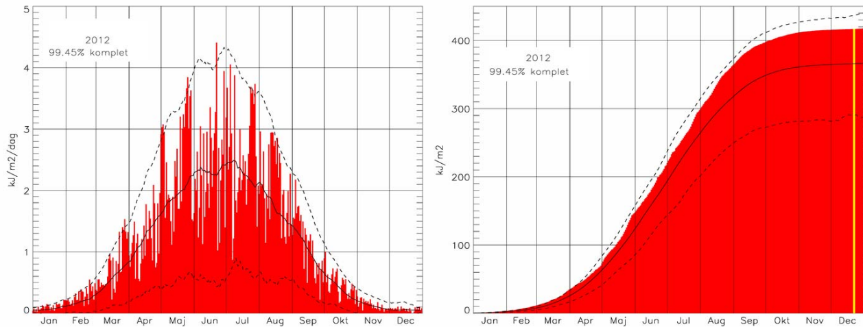
Figur A18e . (Venstre panel) Den dagligt målte totale dosis af hudskadelig UV stråling i 2012 i København i kJ/m 2 /dag. Fuldt optrukken kurve er den tilsvarende middel-dosis for 2000-2010. Øvre og nedre punkterede kurver viser hhv. +2 og -2 standardafvigelser. (Højre panel) Den totale dosis i løbet af året af hudskadelig UV stråling i København i kJ/m 2 . Fuldt optrukken kurve er den tilsvarende middel-dosis. Øvre og nedre punkterede kurver viser hhv. +2 og -2 standardafvigelser.
