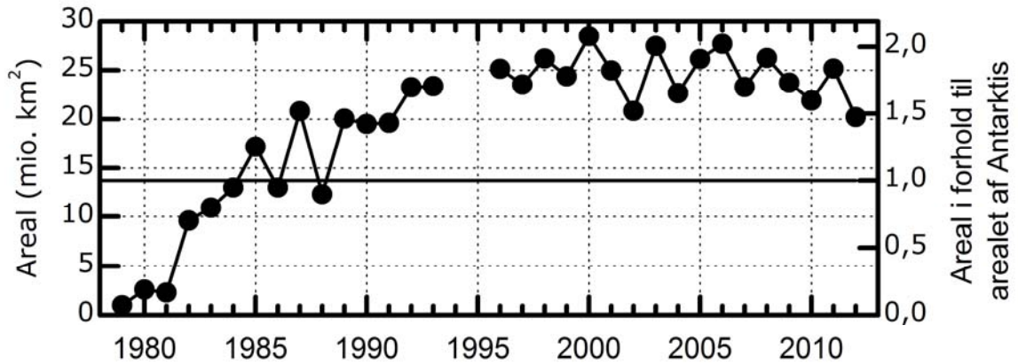
Figur14. Det maksimale areal af det antarktiske ozonhul i perioden 1979-2012.
