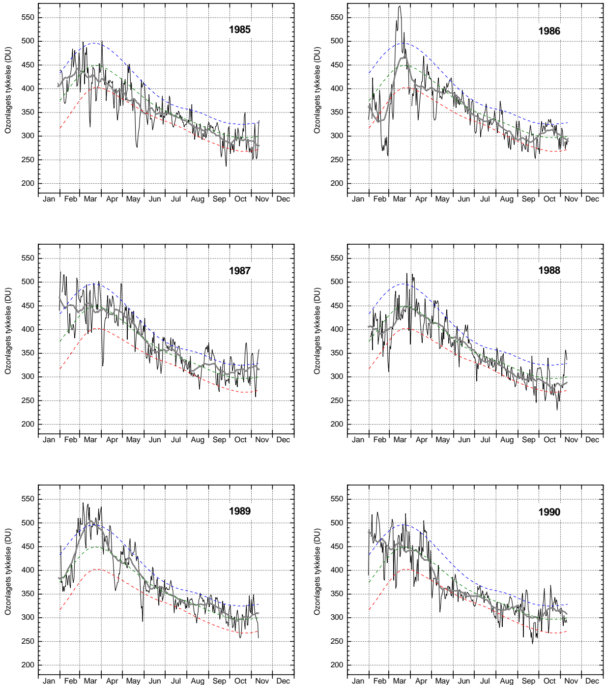
Figur A8. Ozonlagets tykkelse over Kangerlussuaq 1985-1990. Daglige målinger (tynd, sort linje) er fra NASA's TOMS instrument på Nimbus 7 satellitten. Den grønne stiplede linje angiver middelværdien af daglige målinger i 10-års perioden 1979-1988, mens de blå og røde stiplede linjer angiver henholdsvis middelværdien plus (blå) eller minus (rød) en standardafvigelse fra middelværdien. Det betyder, at ca. 2/3 af alle målinger i perioden 1979-1988 ligger mellem den blå og den røde linje. Den tykke grå linje er en 31-dages løbende middelværdi af de daglige målinger.
