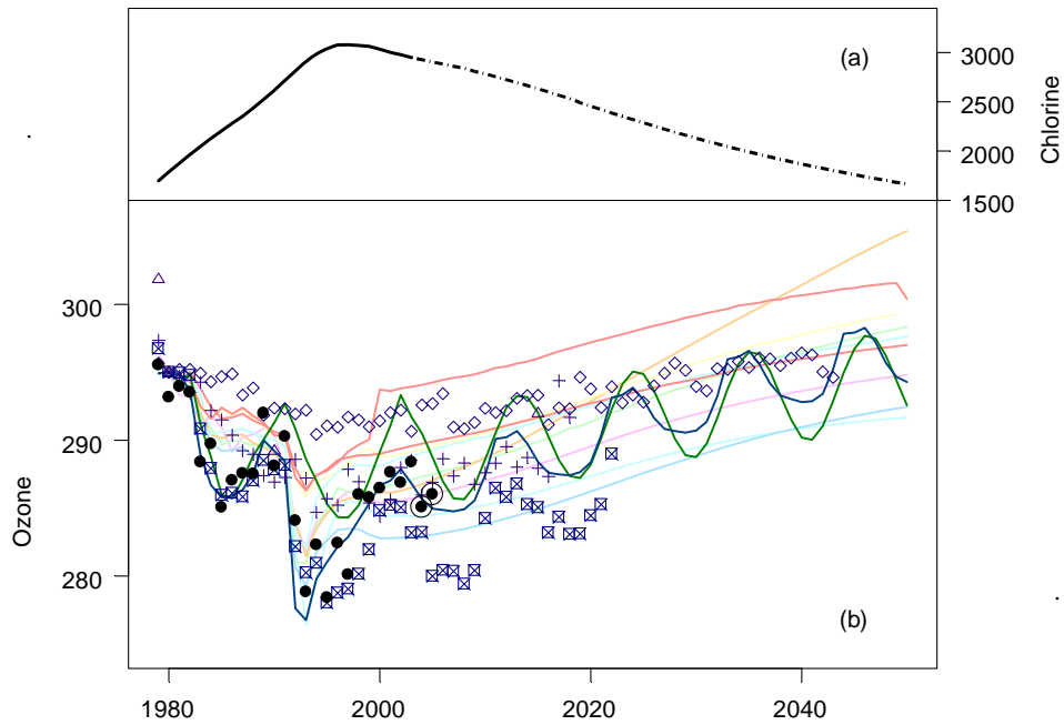
Figur 32. Øverst: Mængden af ozonnedbrydende stoffer som funktion af tiden. Den fuldt optrukne linie baserer sig på målinger, mens den stiplede linie viser den forventede udvikling, hvis Montreal-protokollen med tilføjelser overholdes. Nederst: Modelforudsigelser af fremtidens ozonlag midlet fra 60°S til 60°N. Linierne viser resultaterne fra to-dimensionelle modeller, symbolerne fra tre-dimensionelle modeller, og de sorte prikker er satellitobservationer. De meget lave værdier omkring 1993 skyldes udbruddet af vulkanen Mount Pinatubo på Filippinerne. Figuren er fra Weatherhead og Andersen, 2006.
