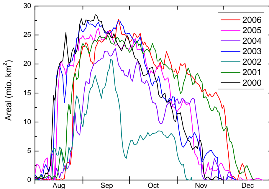
Figur 30. Udviklingen i det antarktiske ozonhuls areal de seneste 7 år.
