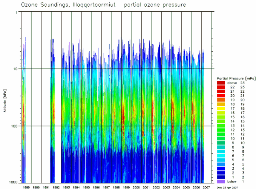
Figur 23. Oversigt over alle ozonsonderinger i Illoqqortoormiut. Figuren viser ozonens partialtryk som funktion af tid og trykhøjde. Se også figur A1 i appendiks 1.
