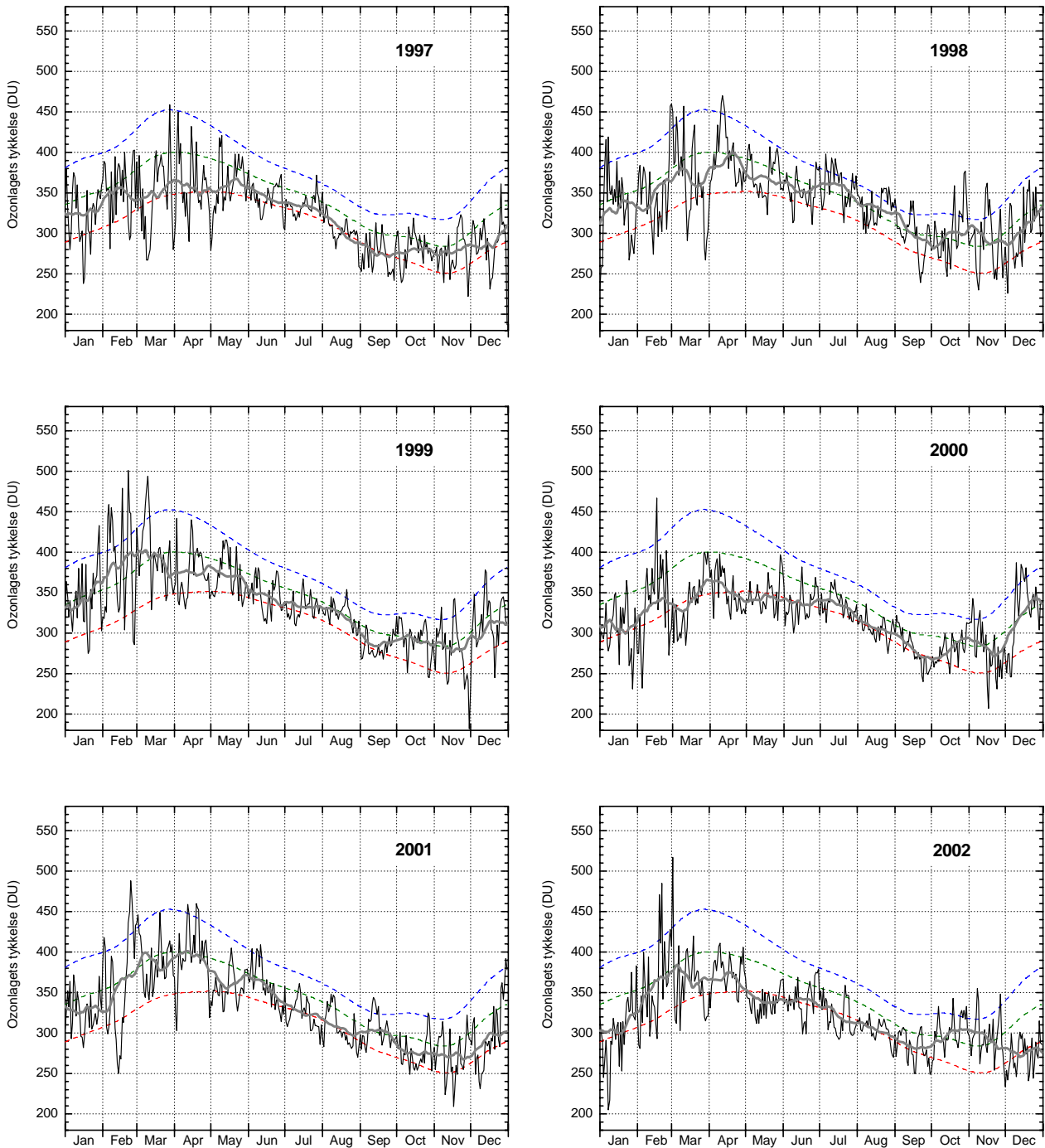
Figur 7. Ozonlagets tykkelse over Danmark 1997-2002. Daglige målinger (tynd, sort linie) er DMI's målinger i København. Den grønne stiplede linie angiver middelværdien af daglige målinger i 10-års perioden 1979-1988, mens de blå og røde stiplede linier angiver henholdsvis middelværdien plus (blå) eller minus (rød) en standardafvigelse fra middelværdien. Det betyder, at ca. 2/3 af alle målinger i perioden 1979-1988 ligger mellem den blå og den røde linie. Den tykke grå linie er en 31-dages løbende middelværdi af de daglige målinger. Forholdsvis stor ozonnedbrydning i den polare stratosfære i vinteren 1999-2000 sætter sine spor med forholdsvis tyndt ozonlag forår og sommer 2000. En forholdsvis varm polar stratosfære i vintrene 1997-1998, 1998-1999, 2000-2001 og 2001-2002 med deraf følgende ringe ozonnedbrydning sætter sine spor i de følgende forår og somre med forholdsvis normalt ozonlag.
