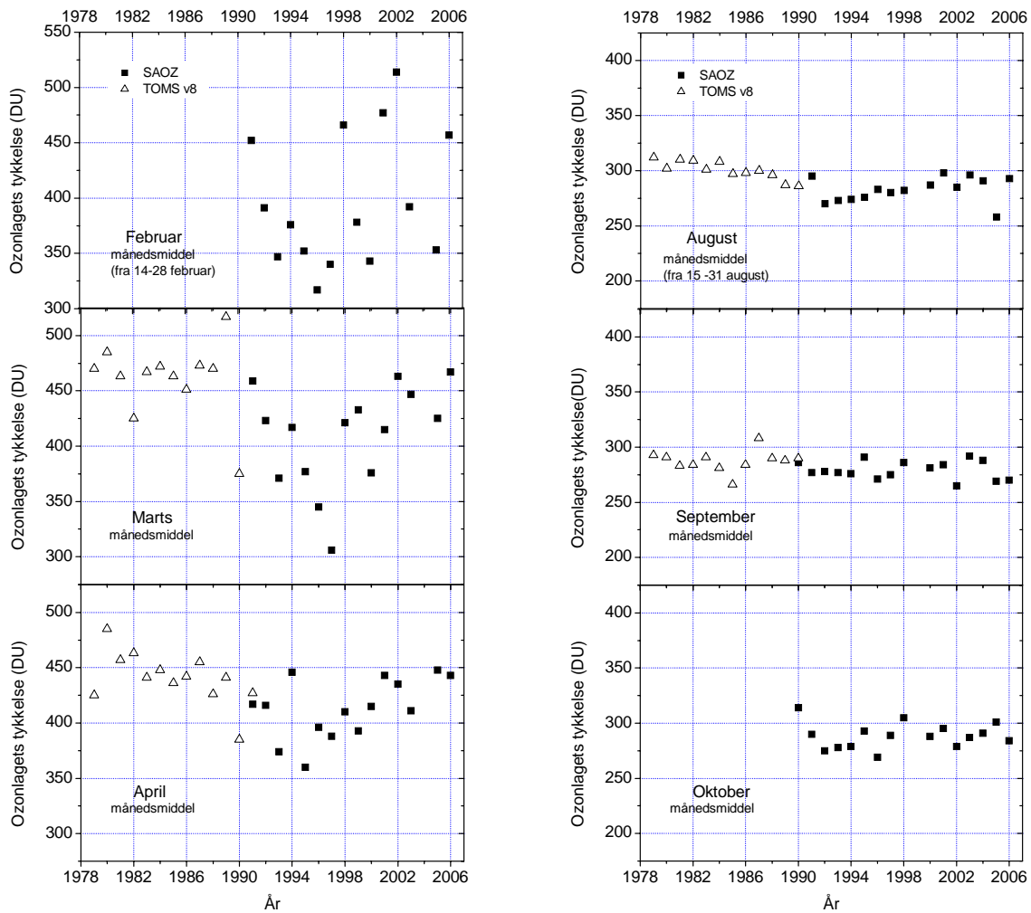
Figur 15. Månedsmidler af ozonlagets tykkelse over Pituffik. Data fra før september 1990 (trekanter) er målinger med NASAS's TOMS-instrument. Data fra og med september 1990 (firkanter) er målinger med DMI's SAOZ-instrument.
