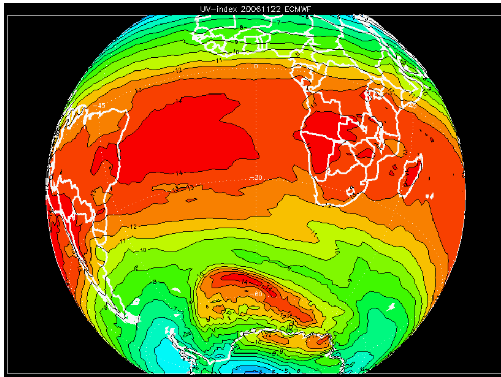
Figur 31. Beregnede UV-indices over det sydlige Atlanterhav 22. november 2006. Bemærk de kraftigt forhøjede UV-niveauer ved 60°S i forbindelse med det antarktiske ozonhul.
