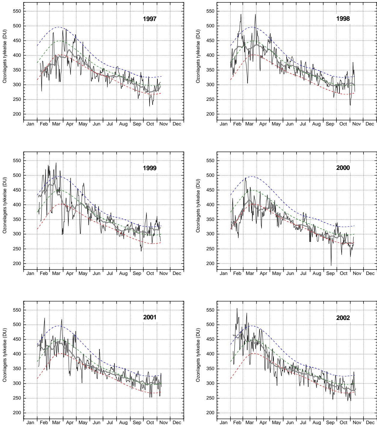
Figur 13. Ozonlagets tykkelse over Kangerlussuaq 1997-2002. Daglige målinger (tynd, sort linie) er DMI's målinger i Kangerlussuaq. Den grønne stiplede linie angiver middelværdien af daglige målinger i 10-års perioden 1979-1988, mens de blå og røde stiplede linier angiver henholdsvis middelværdien plus (blå) eller minus (rød) en standardafvigelse fra middelværdien. Det betyder, at ca. 2/3 af alle målinger i perioden 1979-1988 ligger mellem den blå og den røde linie. Den tykke grå linie er en 31-dages løbende middelværdi af de daglige målinger. Forholdsvis stor ozonnedbrydning ses i den polare stratosfære i vinteren 1999-2000, mens en forholdsvis varm polar stratosfære i vintrene 1997-1998, 1998-1999, 2000-2001 og 2001-2002 medfører ringe ozonnedbrydning.
