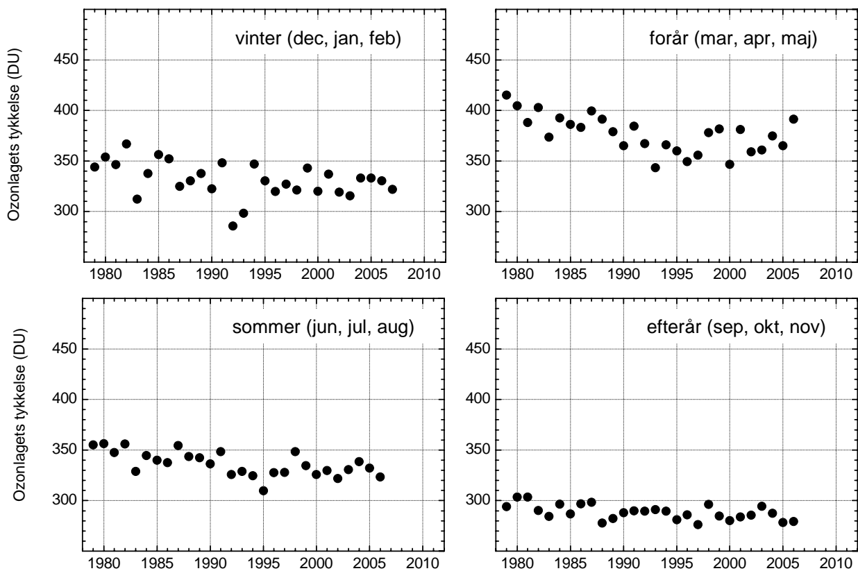
Figur 3. Ozonlagets sæsonmæssige middeltykkelse over Danmark for perioden 1979-2006. Data fra før 1993 er data fra NASA's TOMS-instrument på Nimbus7- satellitten. Data fra og med 1993 er DMI's målinger i København med et Brewer-instrument.
