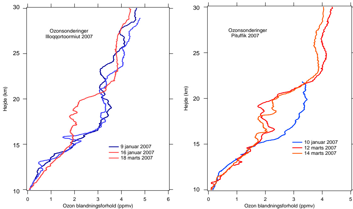
Figur 21. Ozonens blandingsforhold som funktion af højden fra vinteren 2006/2007 målt med ballonbårne ozonsonder fra Illoqqortoormiut og Pituffik. En tydelig nedgang ses i ozonkoncentrationen mellem 15 og 21 km's højde, hvor ozonkoncentrationen falder med mere end en tredjedel i februar og marts.
