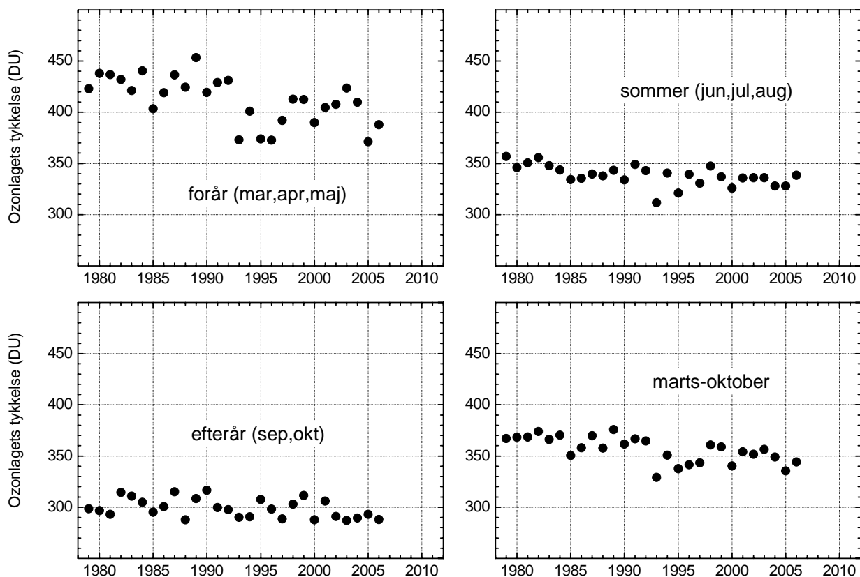
Figur 9. Ozonlagets sæsonmæssige middeltykkelse for Kangerlussuaq for perioden 1979-2006. Der kan kun måles i perioden fra midt i februar til slutningen af oktober. Efterår er derfor begrænset til to måneder, og den årlige middeltykkelse kan ikke bestemmes. En simpel lineær tilpasning af data for perioden 1979-2006 viser en signifikant nedadgående tendens for forår, sommer og hele måleperioden, men ikke for efteråret. Data fra før 1991 er data fra NASA's TOM-instrument på Nimbus7-satellitten, mens data fra og med 1991 er DMI's målinger med et Brewer-instrument.
