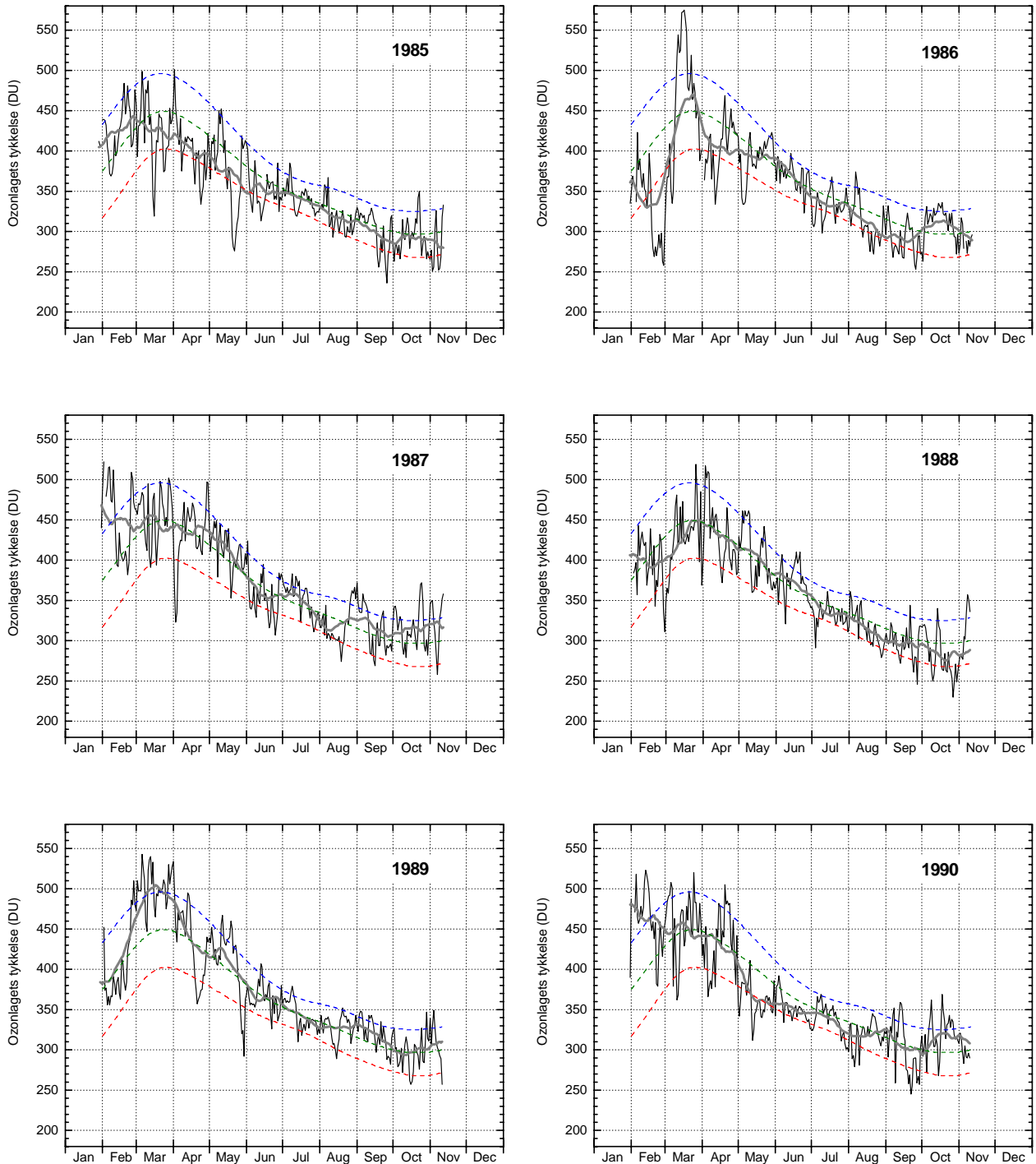
Figur 11. Ozonlagets tykkelse over Kangerlussuaq 1985-1990. Daglige målinger (tynd, sort linie) er fra NASA's TOMS instrument på Nimbus 7 satellitten. Den grønne stiplede linie angiver middelværdien af daglige målinger i 10-års perioden 1979-1988, mens de blå og røde stiplede linier angiver henholdsvis middelværdien plus (blå) eller minus (rød) en standardafvigelse fra middelværdien. Det betyder, at ca. 2/3 af alle målinger i perioden 1979-1988 ligger mellem den blå og den røde linie. Den tykke grå linie er en 31-dages løbende middelværdi af de daglige målinger.
