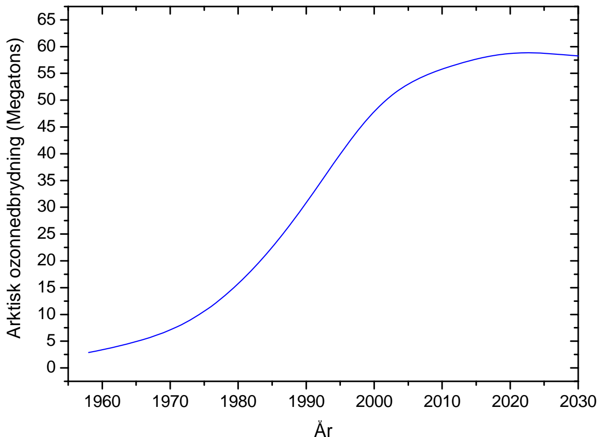
Figur 25: Forudsigelse af den arktiske ozonnedbrydning i de 20% koldeste vintre.
