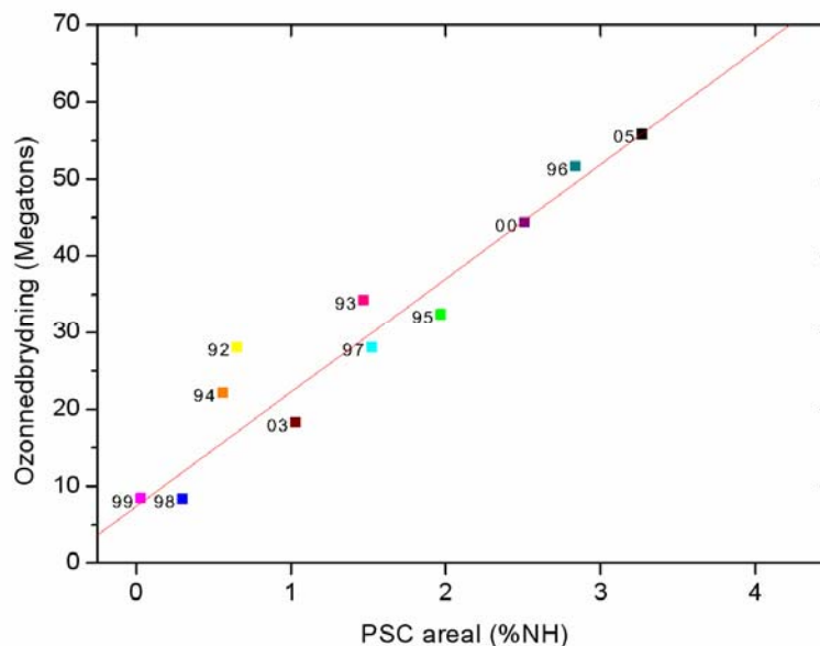
Figur 24. Den maksimale ozonnedbrydning fra januar til marts i den arktiske hvirvel fra 1992-2000 samt 2003 og 2005 som funktion af vinterens gennemsnitlige PSC-areal. Punktet for 1992 er influeret af store mængder af aerosoller fra Pinatubo vulkanens udbrud i juni 1991.
