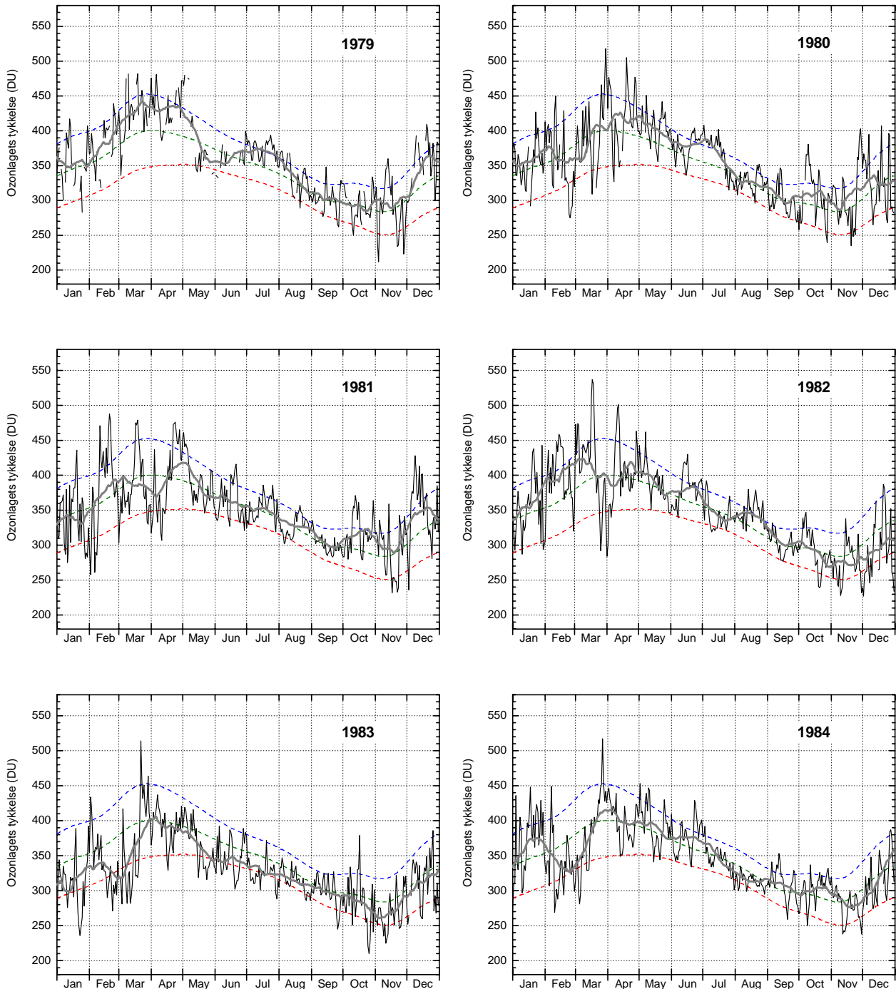
Figur 4. Ozonlagets tykkelse over Danmark 1979-1984. Daglige målinger (tynd, sort linie) er fra NASA's TOMS-instrument på Nimbus7-satellitten. Den grønne stiplede linie angiver middelværdien af daglige målinger i 10-års perioden 1979-1988, mens de blå og røde stiplede linier angiver henholdsvis middelværdien plus (blå) eller minus (rød) en standardafvigelse fra middelværdien. Det betyder, at ca. 2/3 af alle målinger i perioden 1979-1988 ligger mellem den blå og den røde linie. Den tykke grå linie er en 31-dages løbende middelværdi af de daglige målinger. Nogle kraftige vulkanudbrud fandt sted mellem 28. marts og 4. april 1982 (El Chichon, Mexico). Sandsynligvis skyldes det gennemsnitligt noget tynde ozonlag i 1983 dette vulkanudbrud.
