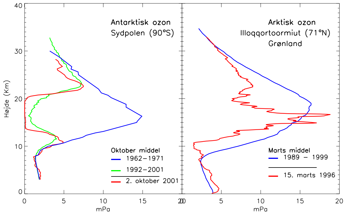
Figur 27. Højdeprofil af ozonnedbrydningen over Antarktis (til venstre) og Arktis (til højre). (WMO Assessment, 2002)
