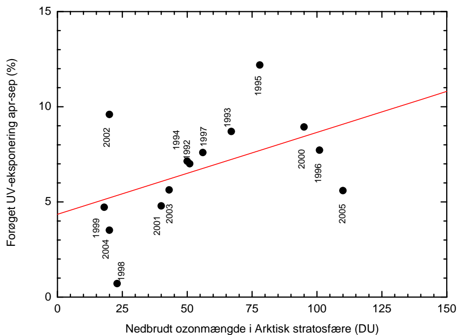
Figur 26. Beregnet sammenhæng mellem den ozonmængde der er nedbrudt i den arktiske stratosfære (14-24 km's højde) i perioden januar-marts og den forøgede UV-eksponering i Danmark i de efterfølgende 5 måneder (april-september). Som referenceniveau er anvendt middelværdien af ozonlagets tykkelse i 10-års perioden 1979-1988 (figur 4 og 5).
