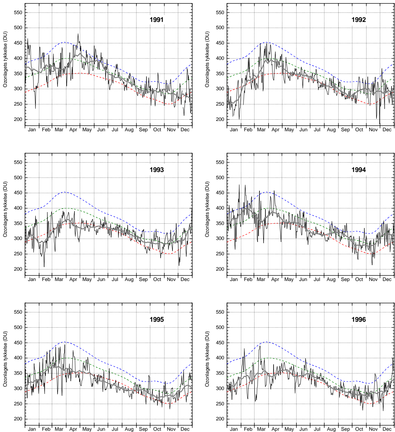
Figur 6. Ozonlagets tykkelse over Danmark 1991-1996. Daglige målinger (tynd, sort linie) frem til maj 1992 er fra NASA's TOMS-instrument på Nimbus7-satellitten, og fra og med juni 1992 DMI's daglige målinger i København. Den grønne stiplede linie angiver middelværdien af daglige målinger i 10-års perioden 1979-1988, mens de blå og røde stiplede linier angiver henholdsvis middelværdien plus (blå) eller minus (rød) en standardafvigelse fra middelværdien. Det betyder, at ca. 2/3 af alle målinger i perioden 1979-1988 ligger mellem den blå og den røde linie. Den tykke grå linie er en 31-dages løbende middelværdi af de daglige målinger. Et kraftigt vulkanudbrud i juni 1991 (Mt. Pinatubo, Filippinerne) påvirker ozonlaget i 1992 og 1993. Forholdsvis stor ozonnedbrydning i den polare stratosfære i vintrene 1991-1992, 1992-1993, 1994-1995 og 1995-1996 sætter sine spor med forholdsvis tyndt ozonlag gennem de efterfølgende somre. I Danmark var sommeren 1995 desuden præget af langvarigt højtryk, hvilket også bidrog til et tyndt ozonlag.
