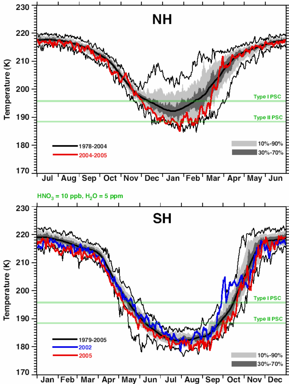
Figur 28. Årlig stratosfærisk temperatur cyklus og variabilitet i Arktis (NH) og Antarktis (SH). De grønne linier angiver temperaturen, hvorunder PSC'er kan dannes. Den sorte kurve angiver middeltemperatur i perioden 1979-2004 (NH) og 1979-2005 (SH) med angivelse af rekordværdier (tynde sorte kurver). Den røde linie angiver udviklingen i Arktis (2004/2005) og Antarktis (2005) og 2002 (blå). Det grå areal angiver det interval, inden for hvilket procentdelen af observationerne falder. (WMO Assessment, 2007).
