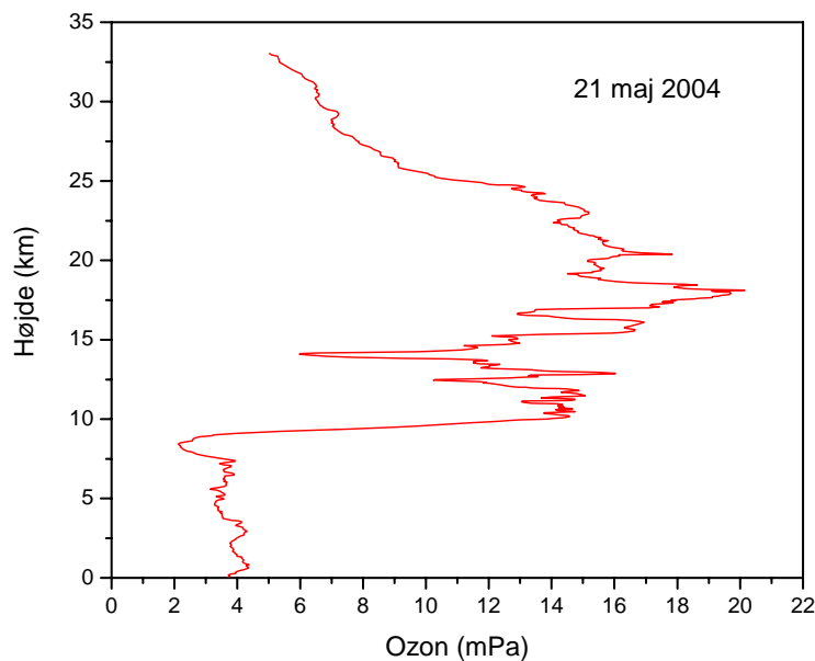
Figur 19. Typisk ozonprofil, målt fra ballon med en elektrokemisk sensor fra Illoqqortoormiut. Figuren viser højdeprofilen af ozonens partialtryk i milli-Pascal.
