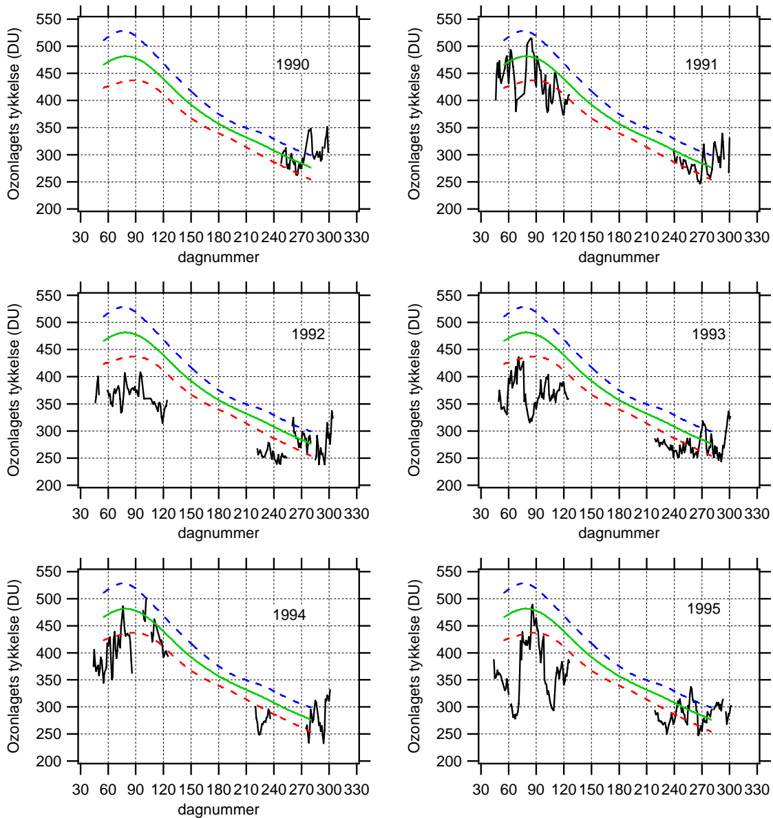
Figur 16. Ozonlagets tykkelse over Pituffik 1990-1995. Daglige målinger (sorte prikker) er DMI's målinger med SAOZ-spektrometeret. Den grønne linie angiver middelværdien af daglige målinger i ti-års perioden 1979-1988 målt med TOMS-instrumentet ombord på Nimbus7-satellitten. De blå og røde stiplede linier angiver plus og minus en standardafvigelse fra middelværdien. Det betyder, at 2/3 af alle målinger i perioden 1979-1988 ligger mellem den blå og den røde linie.
