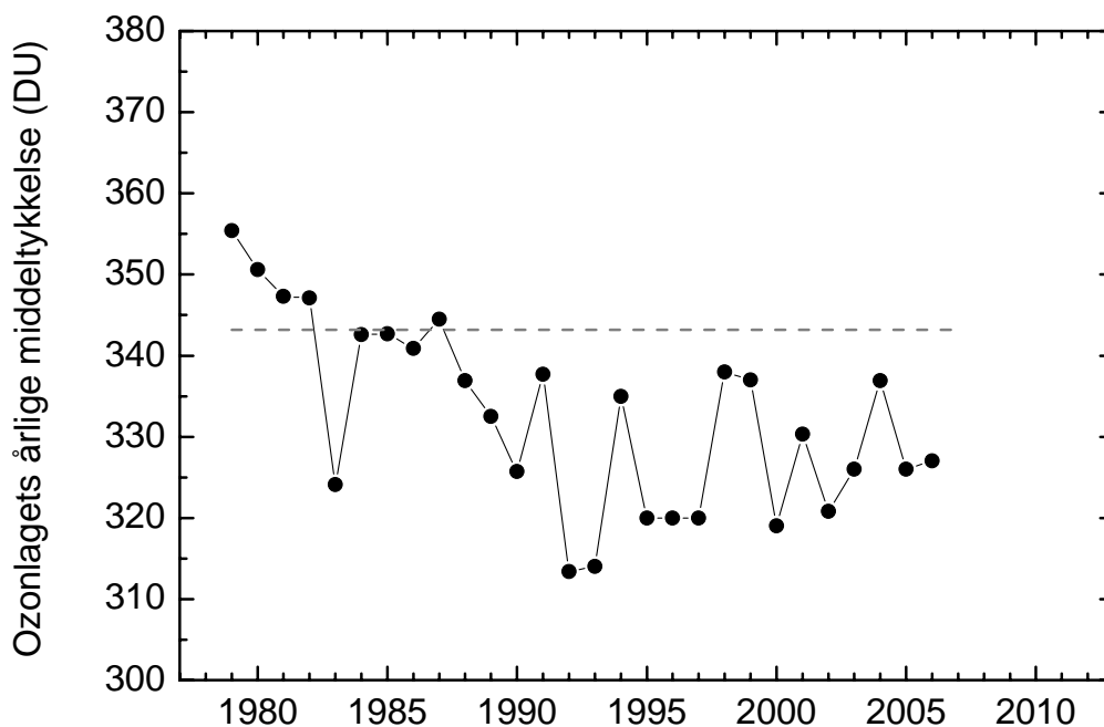
Figur 2. Ozonlagets årlige middeltykkelse over Danmark for perioden 1979-2006. Den gennemsnitlige årlige middelværdi for 10-års perioden 1979-1988 er 344 DU, vist med den stiplede linie. Betragtes alene de sidste 10 års data ses ingen tendens. Data fra før 1993 er data fra NASA's TOMS instrument på Nimbus7- satellitten. Data fra og med 1993 er DMI's målinger i København med et Brewer-instrument.
