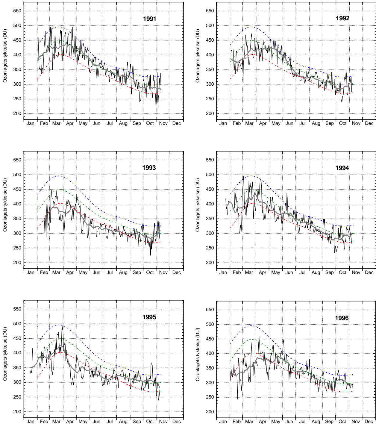
Figur 12. Ozonlagets tykkelse over Kangerlussuaq 1991-1996. Daglige målinger (tynd, sort linie) er DMI's målinger i Kangerlussuaq. Den grønne stiplede linie angiver middelværdien af daglige målinger i 10-års perioden 1979-1988, mens de blå og røde stiplede linier angiver henholdsvis middelværdien plus (blå) eller minus (rød) en standardafvigelse fra middelværdien. Det betyder, at ca. 2/3 af alle målinger i perioden 1979-1988 ligger mellem den blå og den røde linie. Den tykke grå linie er en 31-dages løbende middelværdi af de daglige målinger. Virkningen af et kraftigt vulkanudbrud i juni 1991 (Mt. Pinatubo, Filippinerne) ses i 1992-1993. Forholdsvis stor ozonnedbrydning i den polare stratosfære i vintrene 1991-1992, 1992-1993, 1994-1995 og 1995-1996 sætter sine spor når det polare hvirvelvind er over Kangerlussuaq, hvilket tydeligt ses i februar, marts og april 1996.
