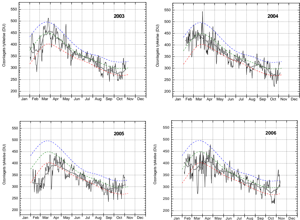
Figur 14. Ozonlagets tykkelse over Kangerlussuaq 2003-2006. Daglige målinger (tynd, sort linie) er DMI's målinger i Kangerlussuaq. Den grønne stiplede linie angiver middelværdien af daglige målinger i 10-års perioden 1979-1988, mens de blå og røde stiplede linier angiver henholdsvis middelværdien plus (blå) eller minus (rød) en standardafvigelse fra middelværdien. Det betyder, at ca. 2/3 af alle målinger i perioden 1979-1988 ligger mellem den blå og den røde linie. Den tykke grå linie er en 31-dages løbende middelværdi af de daglige målinger. En forholdsvis varm polar stratosfære i vintrene 2002-2003 og (især) 2003-2004 medfører ringe ozonnedbrydning.
