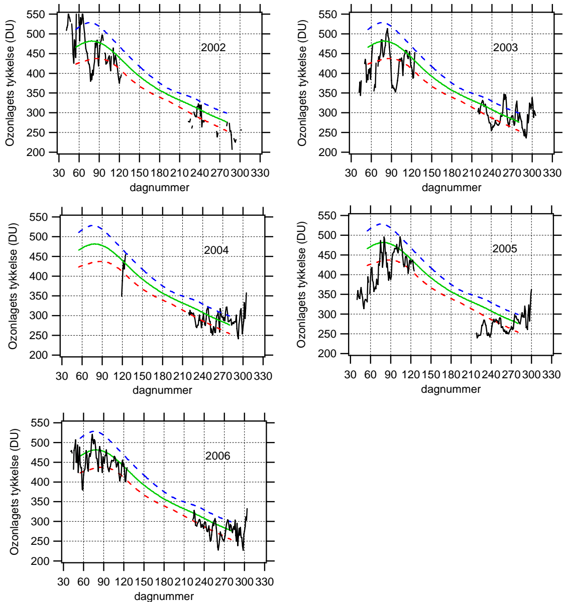
Figur 18. Ozonlagets tykkelse over Pituffik 2002-2006. Daglige målinger (sorte prikker) er DMI's målinger med SAOZ-spektrometeret. Den grønne linie angiver middelværdien af daglige målinger i ti-års perioden 1979-1988 målt med TOMS-instrumentet ombord på Nimbus7-satellitten. De blå og røde stiplede linier angiver plus og minus en standard afvigelse fra middelværdien. Det betyder, at 2/3 af alle målinger i perioden 1979-1988 ligger mellem den blå og den røde linie.
