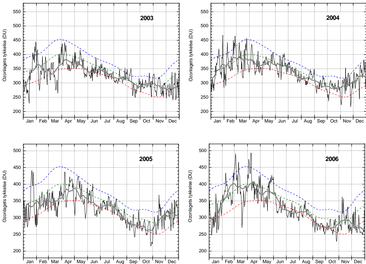
Figur 8. Ozonlagets tykkelse over Danmark 2003-2006. Daglige målinger (tynd, sort linie) er DMI's målinger i København. Den grønne stiplede linie angiver middelværdien af daglige målinger i 10-års perioden 1979-1988, mens de blå og røde stiplede linier angiver henholdsvis middelværdien plus (blå) eller minus (rød) en standardafvigelse fra middelværdien. Det betyder, at ca. 2/3 af alle målinger i perioden 1979-1988 ligger mellem den blå og den røde linie. Den tykke grå linie er en 31-dages løbende middelværdi af de daglige målinger. En forholdsvis varm polar stratosfære i vintrene 2002-2003 og (især) 2003-2004 med deraf følgende ringe ozonnedbrydning sætter sine spor i de følgende forår og somre med forholdsvis normalt ozonlag.
