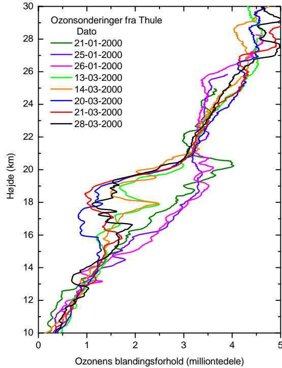
Figur 20. Ozonens blandingsforhold som funktion af højden fra vinteren 1999/2000 målt med ballonbårne ozonsonder fra Pituffik. En tydelig nedgang ses i ozonkoncentrationen mellem 15 og 22 km's højde, hvor ozonen mere end halveres i februar og marts.
