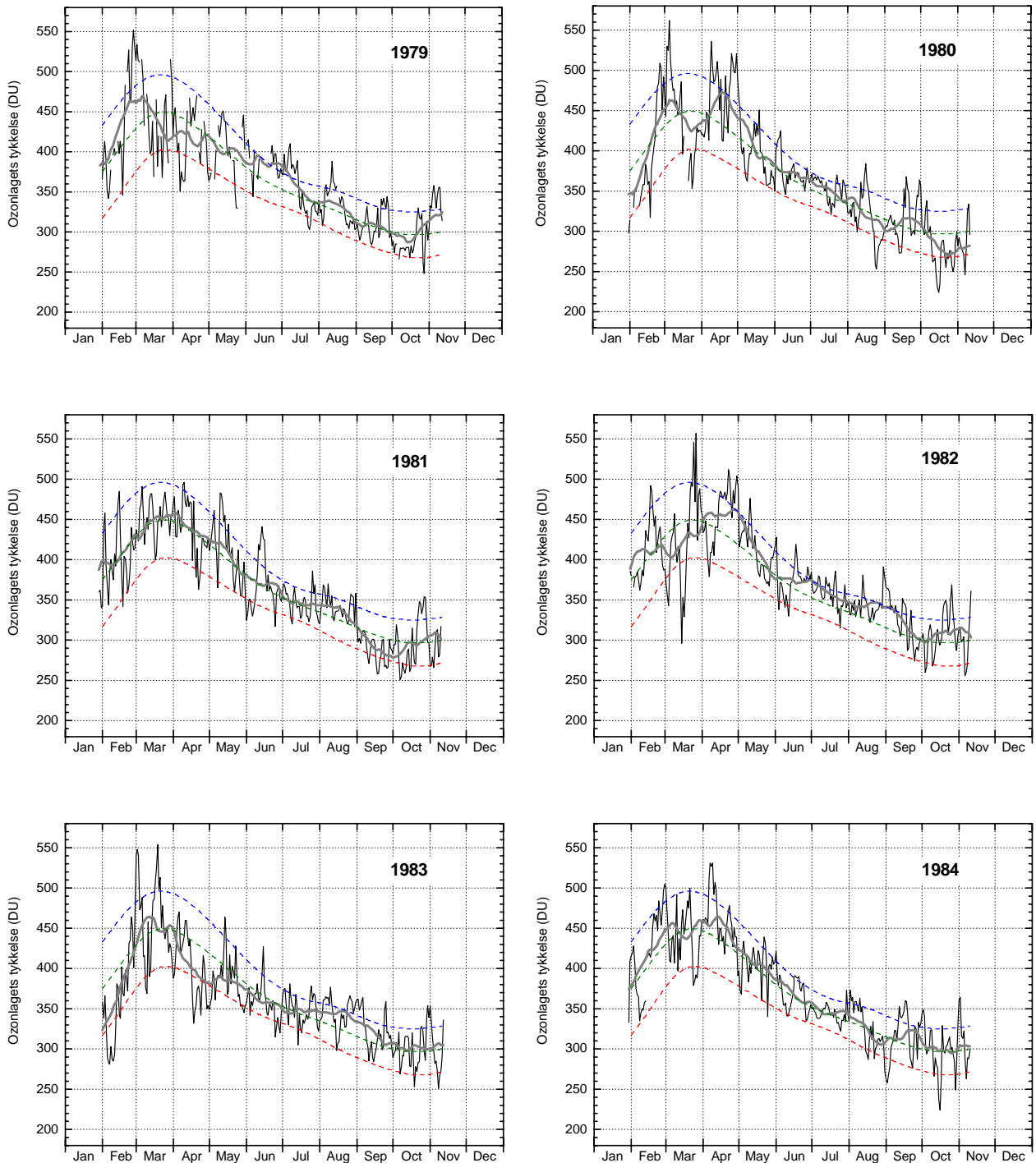
Figur 10. Ozonlagets tykkelse over Kangerlussuaq 1979-1984. Daglige målinger (tynd, sort linie) er fra NASA's TOMS instrument på Nimbus7-satellitten. Den grønne stiplede linie angiver middelværdien af daglige målinger i 10-års perioden 1979-1988, mens de blå og røde stiplede linier angiver henholdsvis middelværdien plus (blå) eller minus (rød) en standardafvigelse fra middelværdien. Det betyder, at ca. 2/3 af alle målinger i perioden 1979-1988 ligger mellem den blå og den røde linie. Den tykke grå linie er en 31-dages løbende middelværdi af de daglige målinger.
