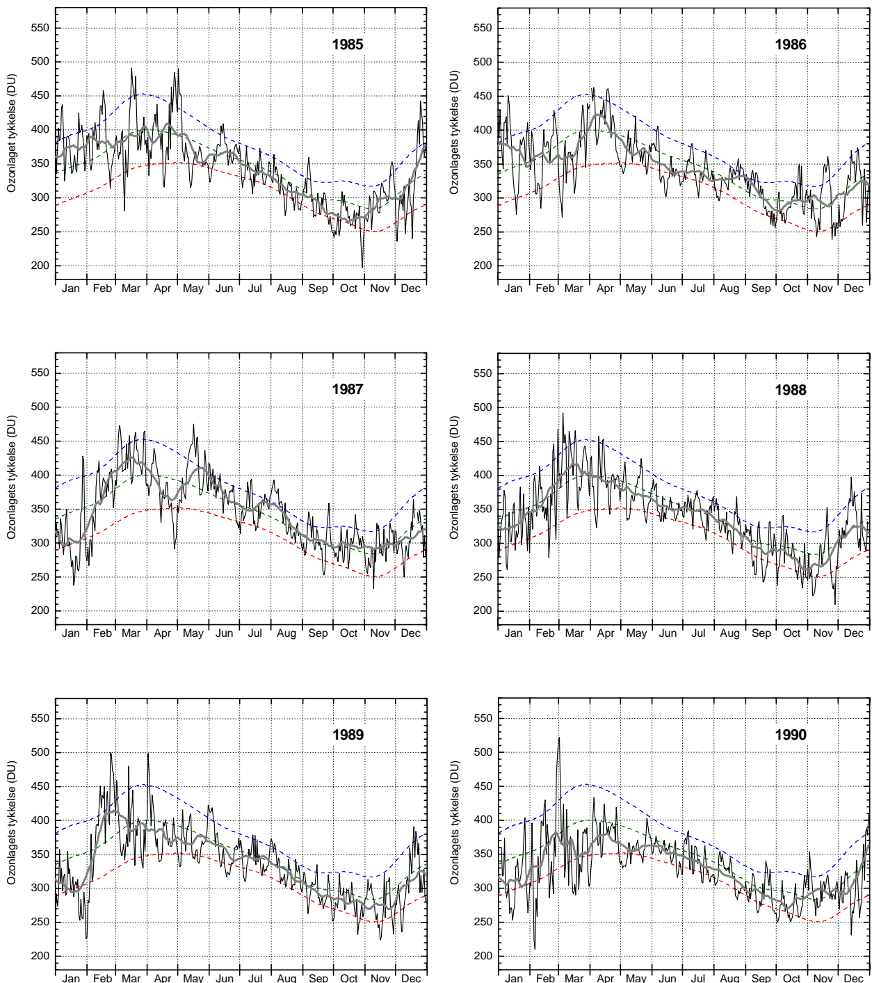
Figur 5. Ozonlagets tykkelse over Danmark 1985-1990. Daglige målinger (tynd, sort linie) er fra NASA's TOMS-instrument på Nimbus7-satellitten. Den grønne stiplede linie angiver middelværdien af daglige målinger i 10-års perioden 1979-1988, mens de blå og røde stiplede linier angiver henholdsvis middelværdien plus (blå) eller minus (rød) en standardafvigelse fra middelværdien. Det betyder, at ca. 2/3 af alle målinger i perioden 1979-1988 ligger mellem den blå og den røde linie. Den tykke grå linie er en 31-dages løbende middelværdi af de daglige målinger.
