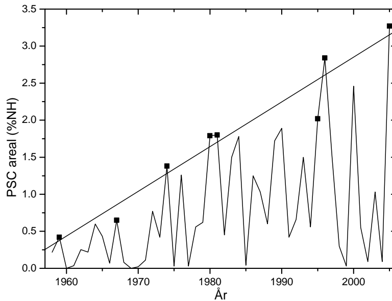
Figur 23. Det gennemsnitlige areal af polar-stratosfæriske skyer i procent af den nordlige halvkugles areal siden 1958. Vintrene med de største PSC-arealer er markeret med kvadrater og danner grundlaget for regressionslinien.
