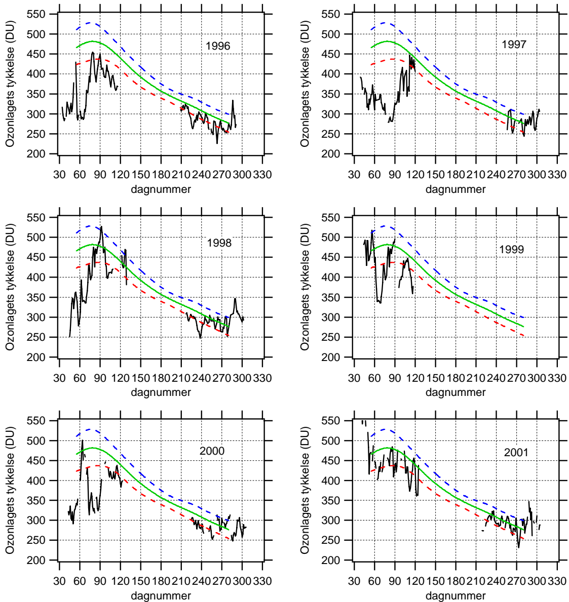
Figur 17. Ozonlagets tykkelse over Pituffik 1996-2001. Daglige målinger (sorte prikker) er DMI's målinger med SAOZ-spektrometeret. Den grønne linie angiver middelværdien af daglige målinger i ti-års perioden 1979-1988 målt med TOMS-instrumentet ombord på Nimbus7-satellitten. De blå og røde stiplede linier angiver plus og minus en standardafvigelse fra middelværdien. Det betyder, at 2/3 af alle målinger i perioden 1979-1988 ligger mellem den blå og den røde linie.
