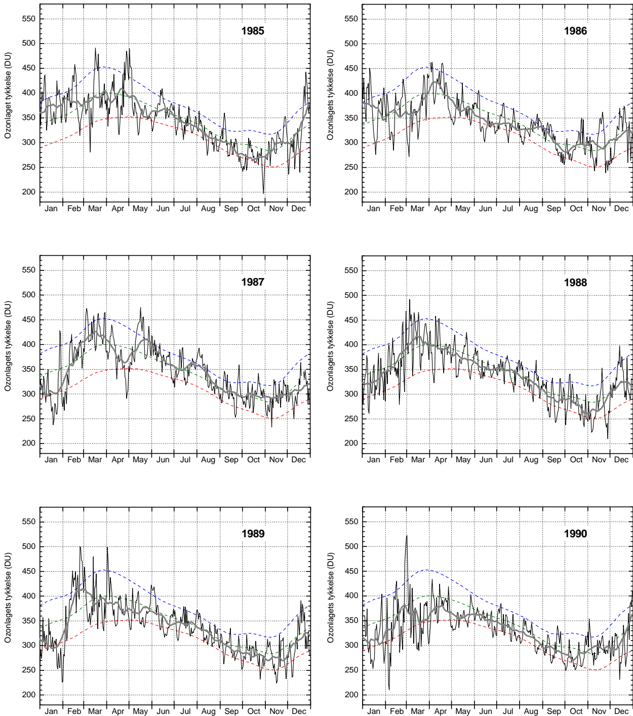
Figur A1b. Ozonlagets tykkelse over Danmark 1985-1990. Daglige målinger (tynd, sort linje) er fra NASA's TOMS-instrument på Nimbus7-satellitten. Den grønne stiplede linje angiver middelværdien af daglige målinger i 10-års perioden 1979-1988, mens de blå og røde stiplede linjer angiver henholdsvis middelværdien plus (blå) eller minus (rød) en standardafvigelse fra middelværdien. Det betyder, at ca. 2/3 af alle målinger i perioden 1979-1988 ligger mellem den blå og den røde linje. Den tykke grå linje er en 31-dages løbende middelværdi af de daglige målinger.
