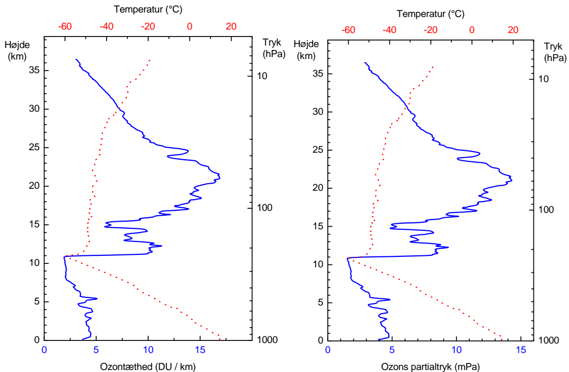
Figur B1. Ozon- og temperaturprofil fra Illoqqortoormiut (Scoresbysund), Grønland, den 13. juli 1994 målt med en ozonsonde. Instrumentet måler ozonkoncentrationen under opstigningen. Koncentrationen kan angives på flere måder: f.eks. som antal ozonmolekyler pr. kubikmeter luft, som antal Dobson-enheder pr. km. (som i figuren til venstre), eller som ozonens partialtryk i mPa (millipascal) (som i figuren til højre). Ozonkoncentrationen er vist med den fuldt optrukne blå kurve, mens temperaturen er vist med den stiplede røde kurve. Skala for ozon er nederst, for temperatur øverst.
