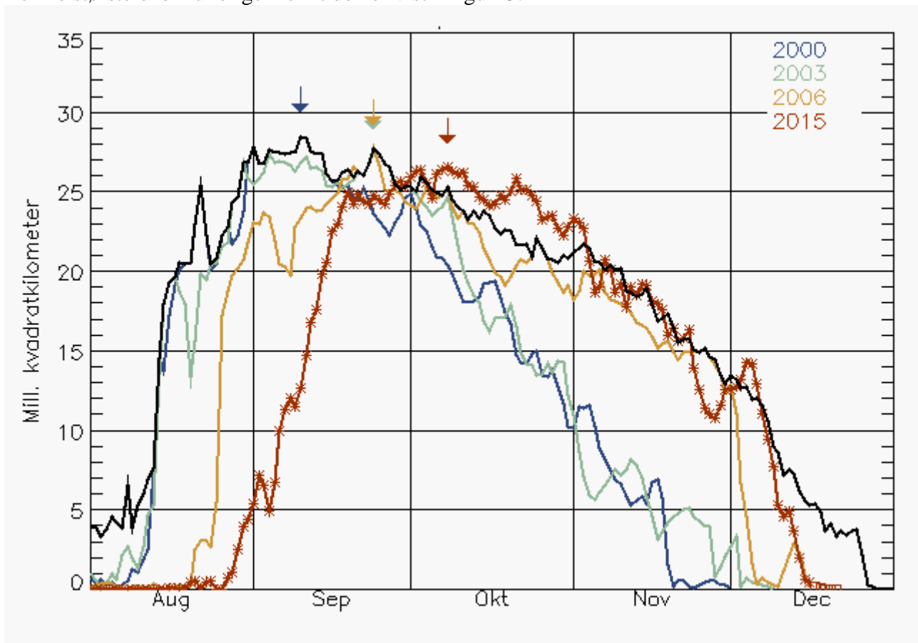
Figur 15. De fire største ozonhuller gennem tiden. Sort kurve: den maksimale størrelse af ozonhullet i perioden 1980-2014. Farvede kurver for hvert af årene 2000,2003,2006 og 2015, maksimum angivet ved pile]
