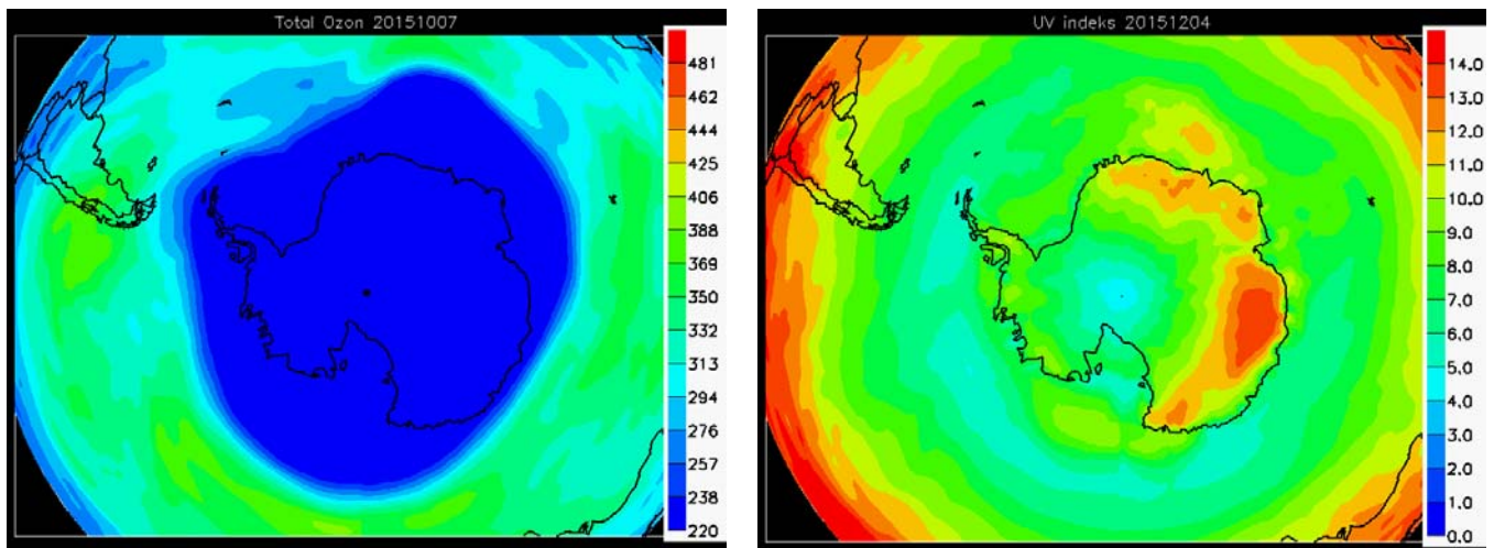
Figur 16. Beregnede UV-indices over det sydlige Amerika 7.oktober 2015 (højre panel) i forbindelse med det antarktiske ozonhul (venstre panel, DU).
