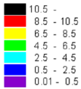
Figur A4e. Areal af den nordlige halvkugle dækket af PSC'ere i højdeinterval 350-675 K potentiel temperatur, svarende til ca. 14-26 km gennem vintren 2014-2016.
