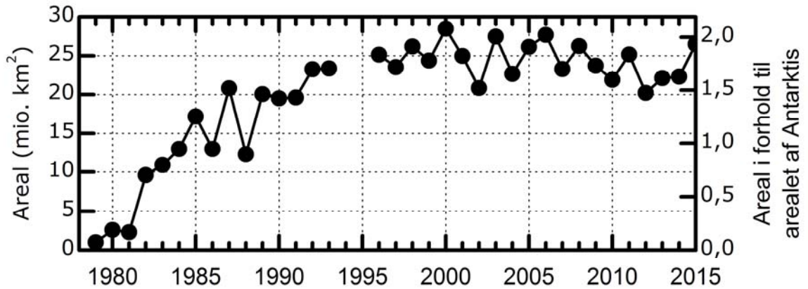
Figur14. Det maksimale areal af det antarktiske ozonhul i perioden 1979-2015.
