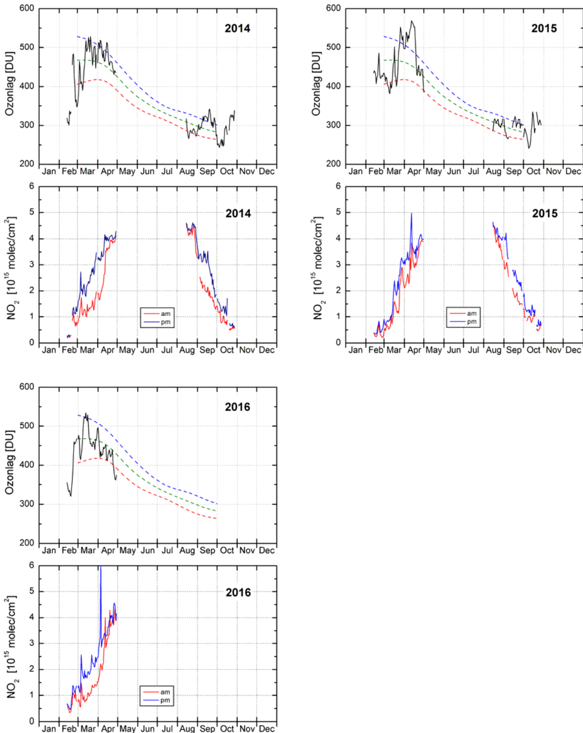
Figur A3g. Daglige målinger af ozonlagets tykkelse samt stratosfærisk NO 2 over Pituffik 2014-2016. For ozonlaget angiver den grønne linie middelværdien af daglige målinger i ti-års perioden 1979-1988 målt med TOMS-instrumentet på Nimbus7-satellitten mens de blå og røde stiplede linjer angiver hhv. plus én og minus én standardafvigelse fra middelværdien. Det betyder, at 2/3 af alle målinger i perioden 1979-1988 ligger mellem den blå og den røde linje. NO 2 målingerne viser hhv. morgen- (solopgang - am) og aftenværdier (solnedgang - pm).
