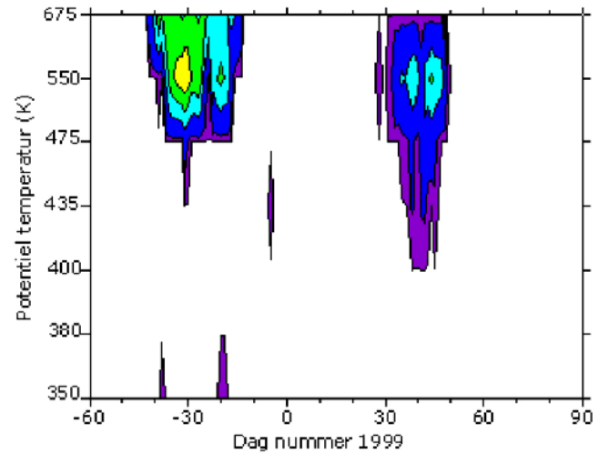
Figur A4b. Areal af den nordlige halvkugle dækket af PSC'ere i højdeinterval 350-675 K potentiel temperatur, svarende til ca. 14-26 km gennem vintrene 1999-2003.
