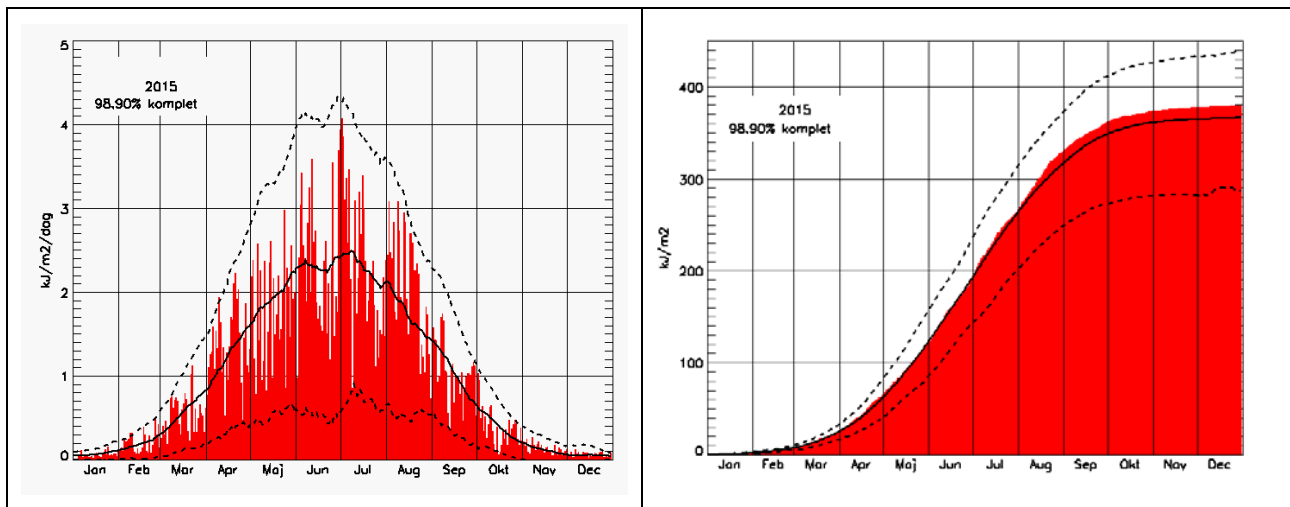
Figur 11 . (Venstre panel) Den dagligt målte totale dosis af hudskadelig UV stråling i 2015 i København i kJ/m 2 /dag. Fuldt optrukken kurve er den tilsvarende middel-dosis for 2000-2010. Øvre og nedre punkterede kurver viser hhv. +2 og -2 standardafvigelser. (Højre panel) Den totale dosis i løbet af året af hudskadelig UV stråling i 2015 i København i kJ/m 2 . Fuldt optrukken kurve er den tilsvarende middel-dosis for 2000-2010. Øvre og nedre punkterede kurver viser hhv. +2 og -2 standardafvigelser.
