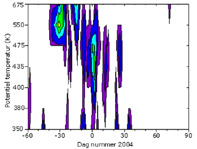
Figur A4c. Areal af den nordlige halvkugle dækket af PSC'ere i højdeinterval 350-675 K potentiel temperatur, svarende til ca. 14-26 km gennem vintrene 2004-2008.
