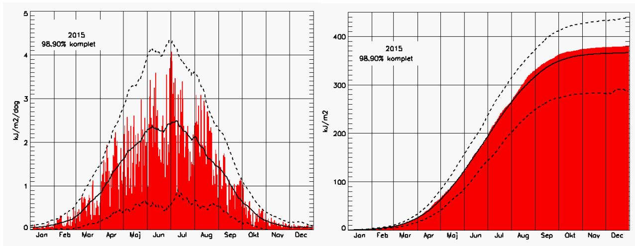
Figur A5f. (Venstre panel) Den dagligt målte totale dosis af hudskadelig UV stråling i 2015 i København i kJ/m 2 /dag. Fuldt optrukken kurve er den tilsvarende middel-dosis for 2000-2010. Øvre og nedre punkterede kurver viser hhv. +2 og -2 standardafvigelser. (Højre panel) Den totale dosis i løbet af året af hudskadelig UV stråling i København i kJ/m 2 . Fuldt optrukken kurve er den tilsvarende middel-dosis. Øvre og nedre punkterede kurver viser hhv. +2 og -2 standardafvigelser.
