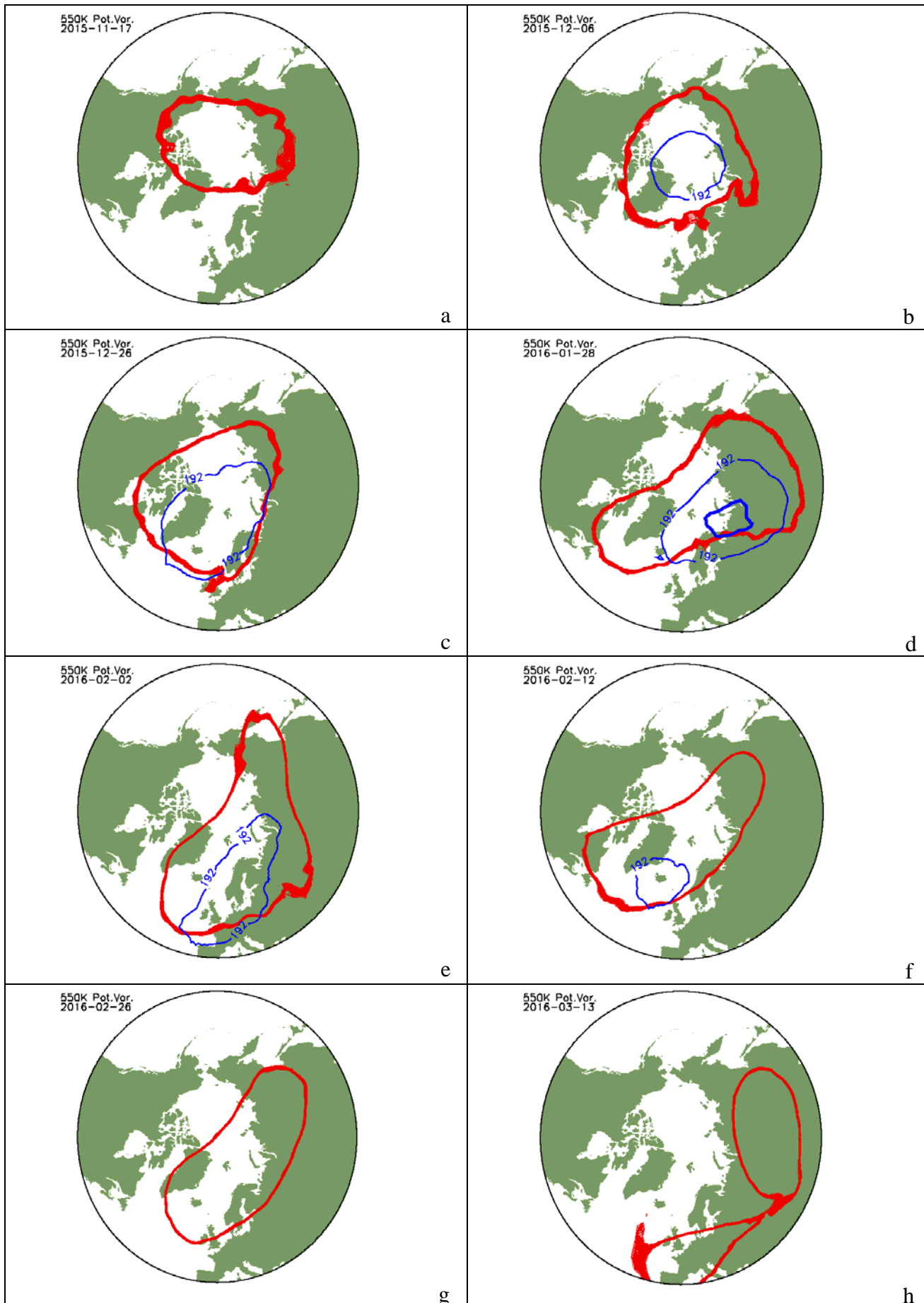
Figur 7. Røde konturlinjer viser grænsen for den polare vortex i 550 K potentieltemperaturshøjde, svarende til ca. 23 km, i perioden 17. november 2015 – 13. marts 2016. Blå konturlinjer viser isothermen for dannelse af type 1 polar-stratosfæriske skyer.
